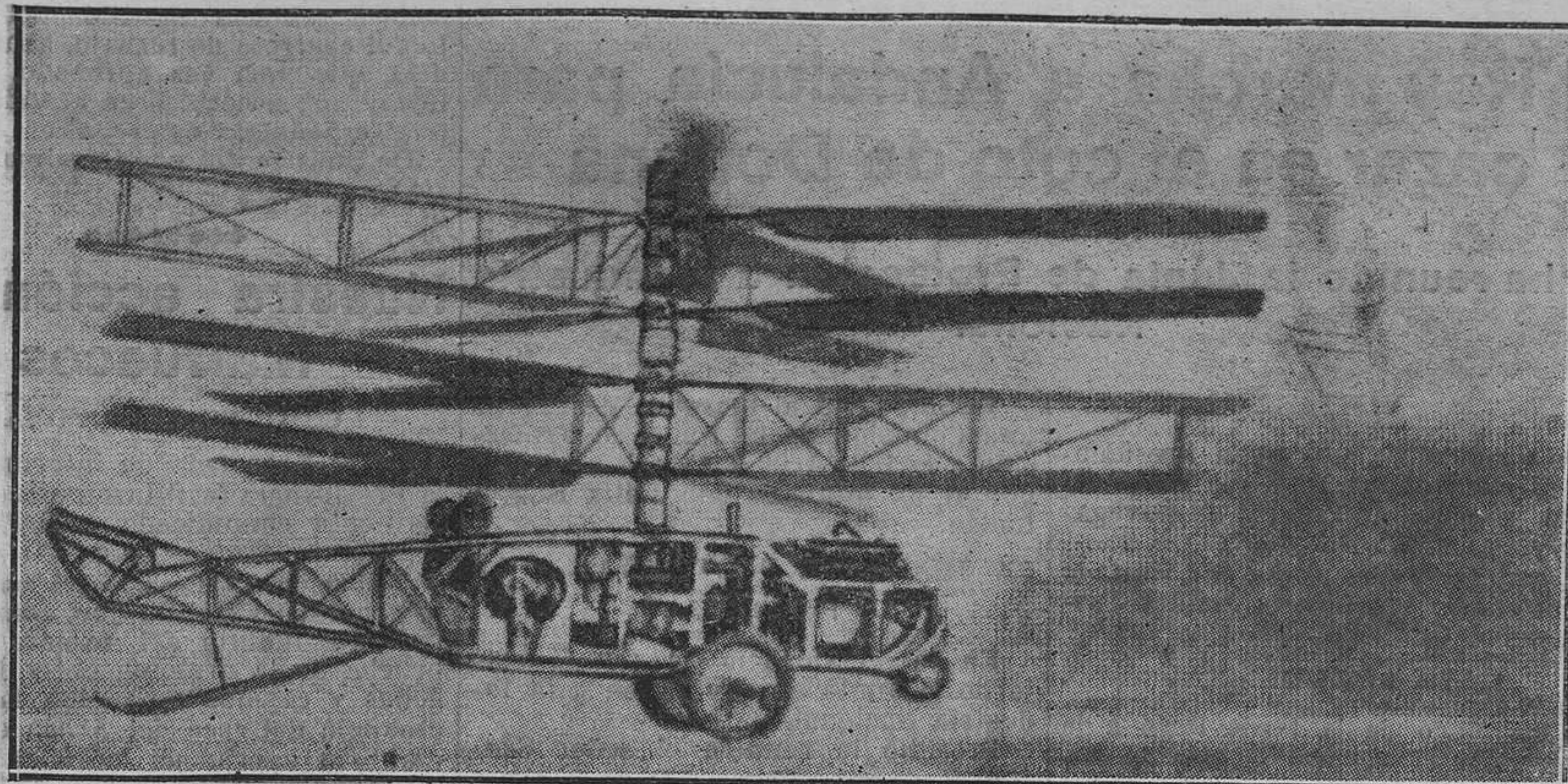
En el aeródromo de Yssy-les-Moulineaux (Francia), el ingeniero español señor Pescara, con un nuevo helicóptero de su invención, ha establecido el record mundial de duración y de distancia. Voló ocho minutos, trece segundos, cuatro quintos. Recorrió 1.160 metros. Esta tentativa, con ser tan feliz, no ha bastado para ganar el premio de 10.000 francos del Aero Club.
