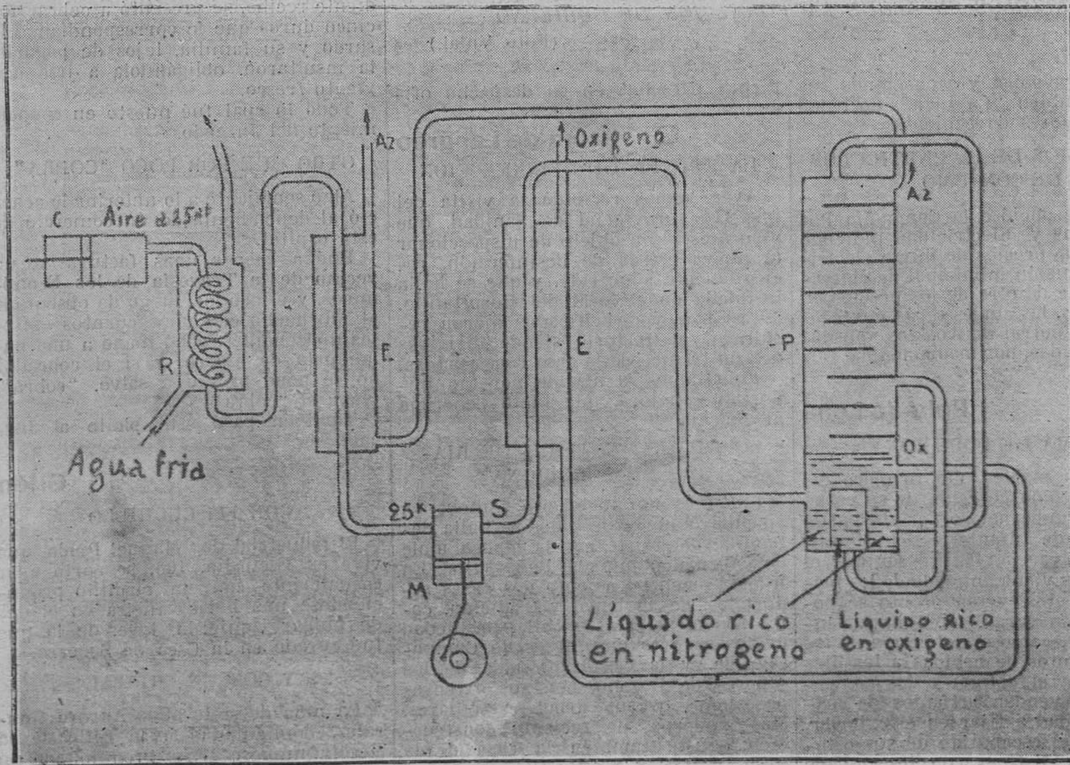
APARATO PARA LA FABRICACION Y DESTILACION DE AIRE LIQUIDO
