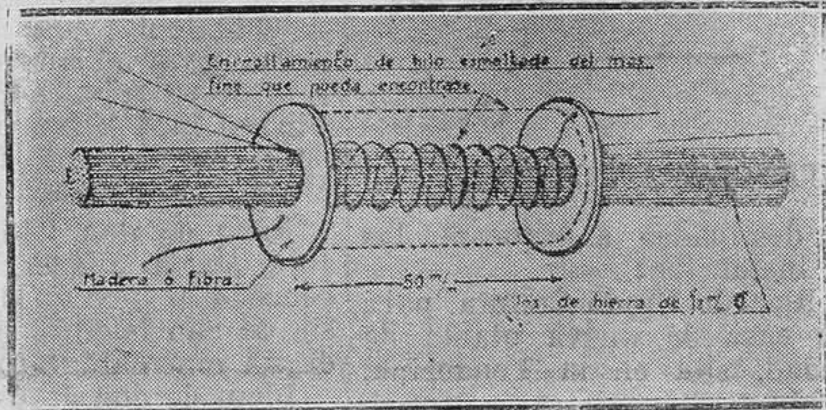
Fig. 4.-Disposición del enrollamiento.
