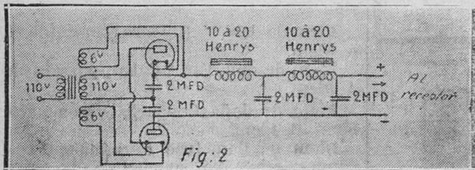
Fig. 2.-Modo de averiguar los polos.
