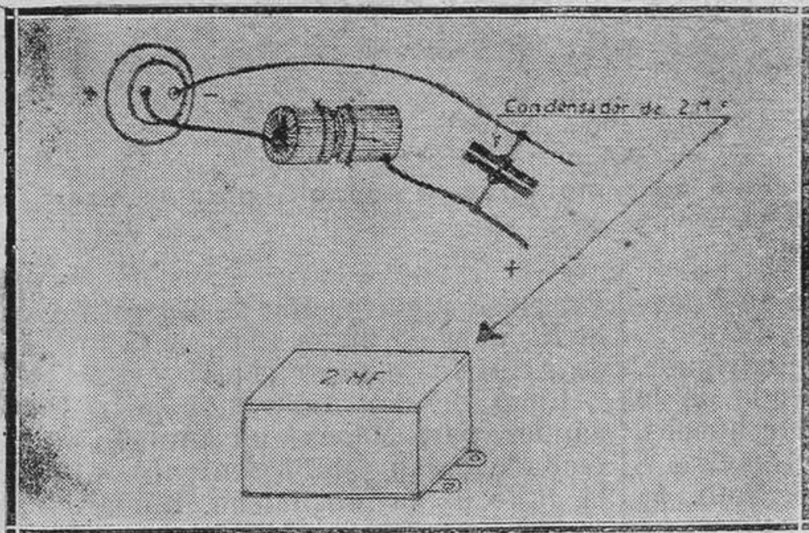
Figura 1.-Principio del esquema.
