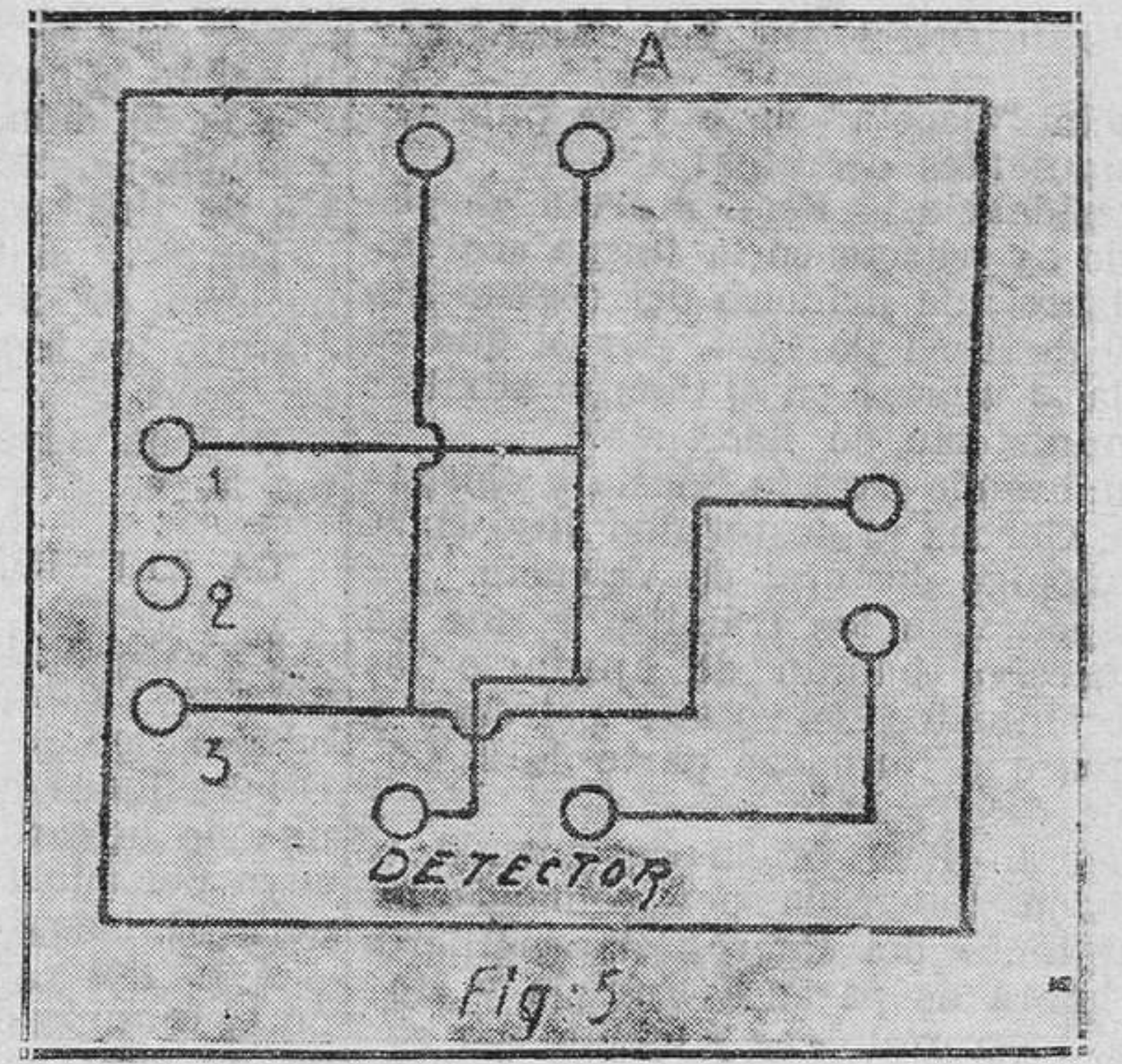
Figura 5.-Esquema de conexiones de la placa de ebonita.
