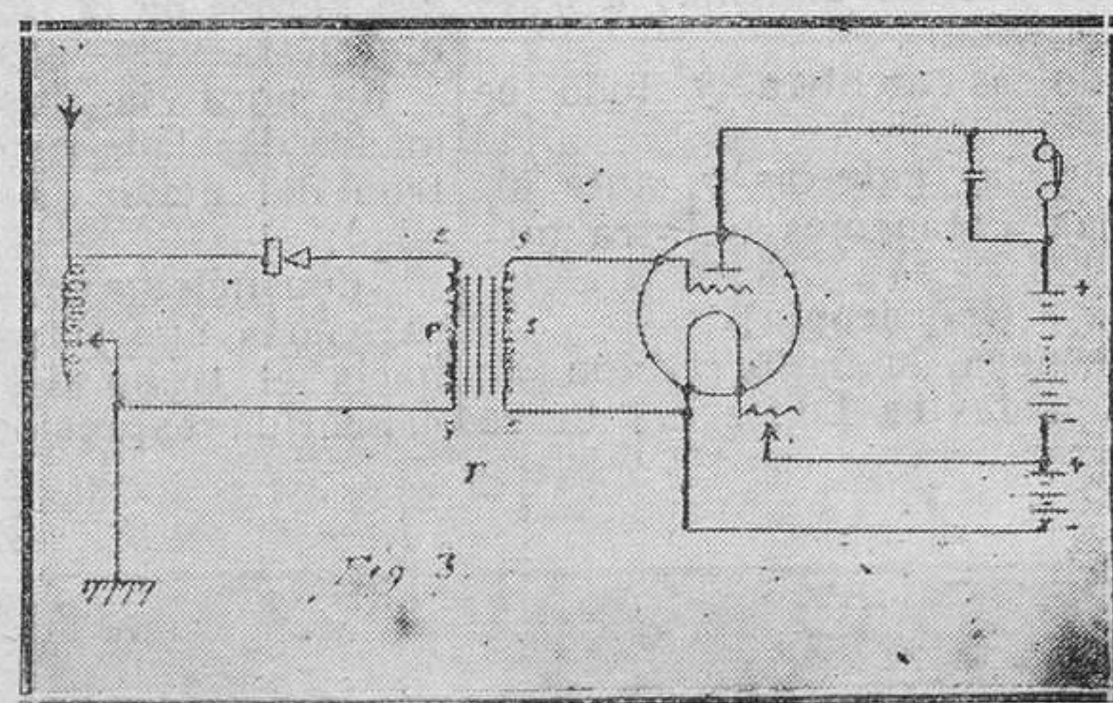
Figura 3.-Amplificador con transformador en baja frecuencia.
