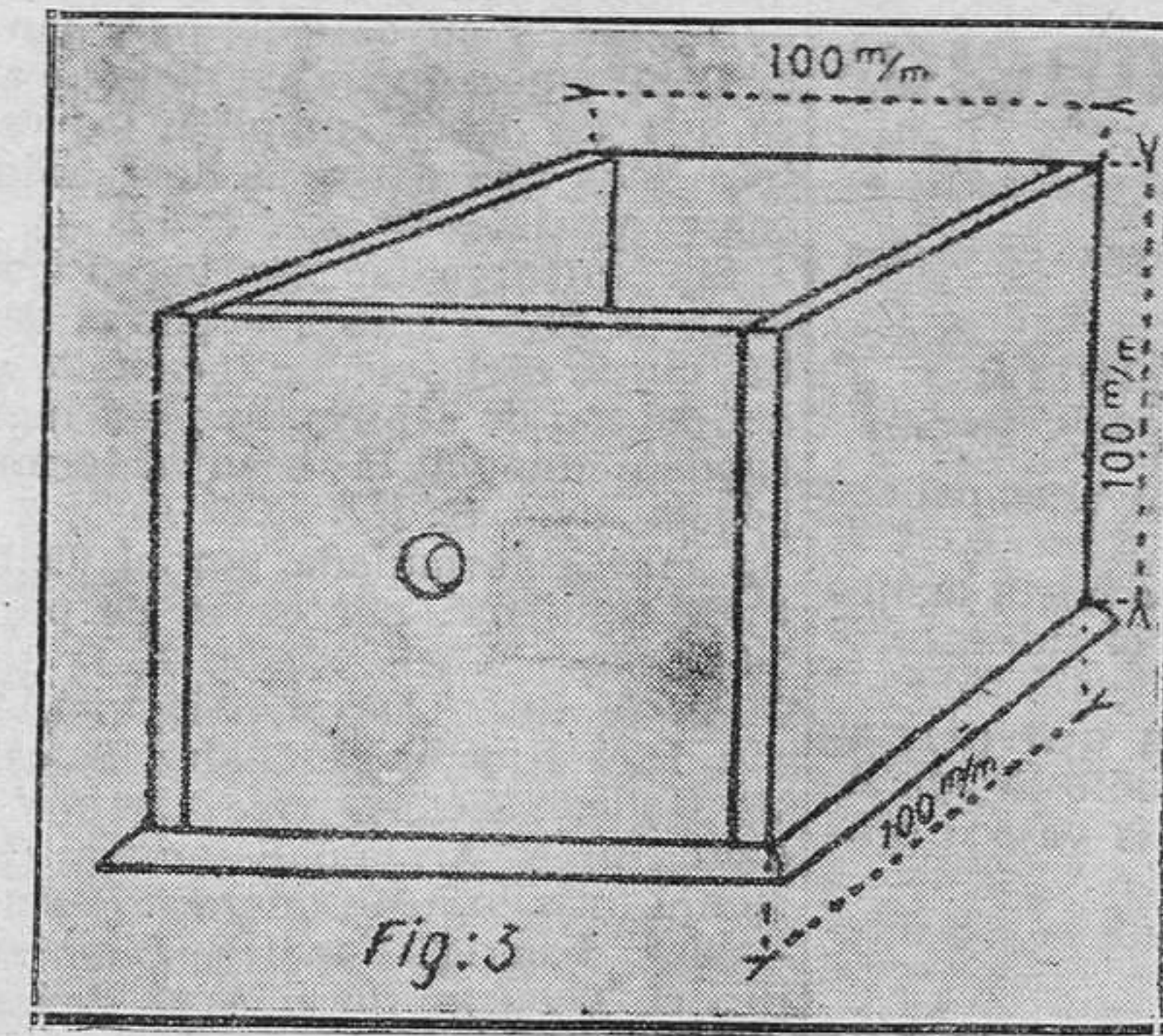
Figura 3.-Dimensiones de la caja.
