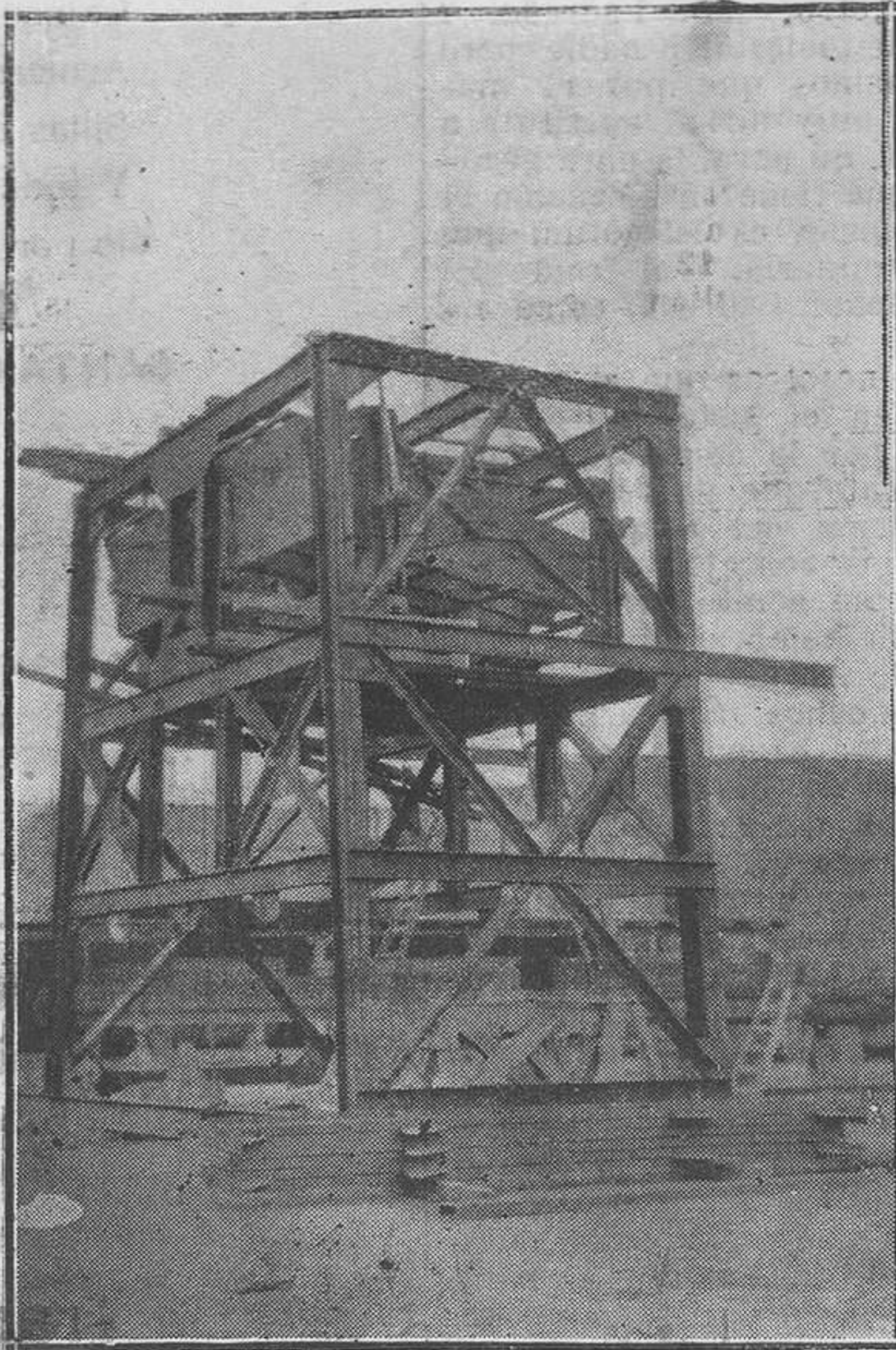
Cribadora de siete metros de altura, del nuevo lavadero que construye "Huileras de Turón".
