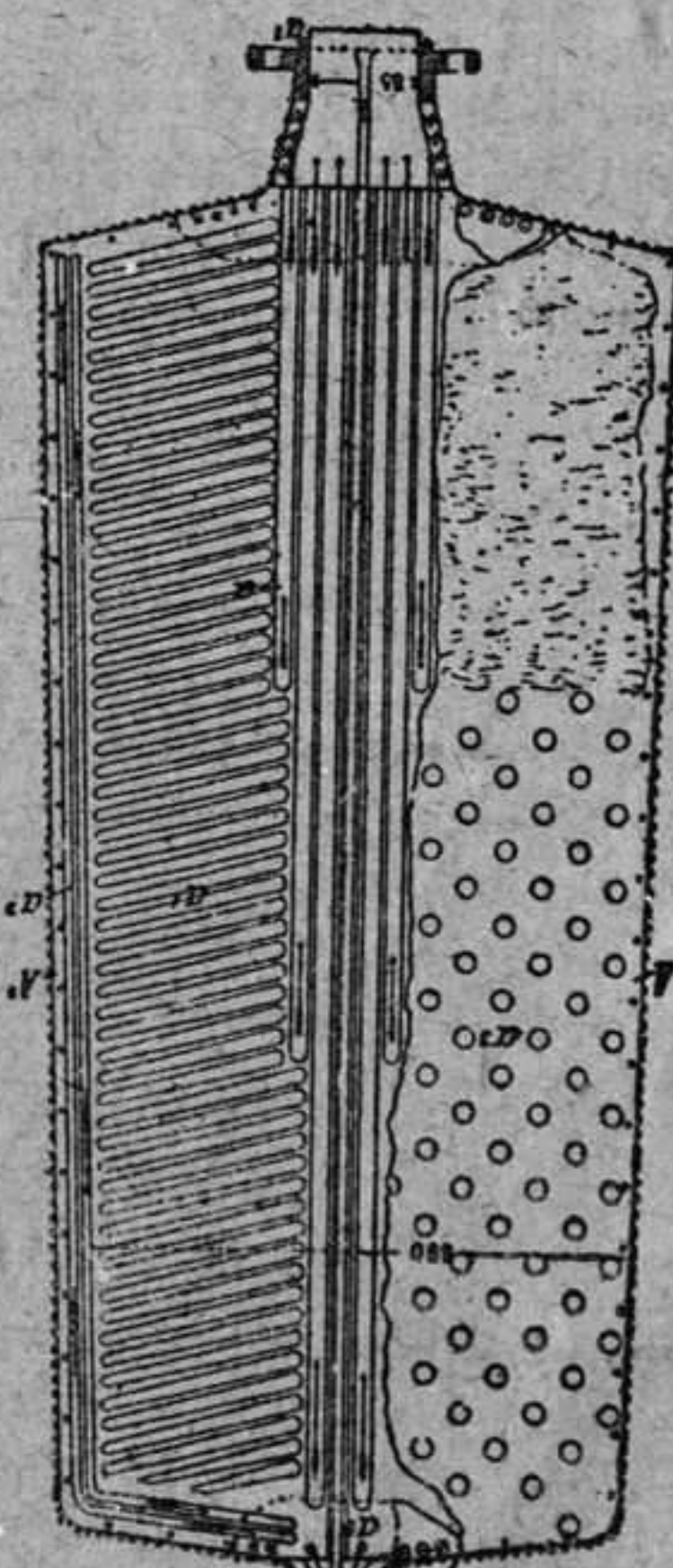
Hoja ó paleta filtradora
