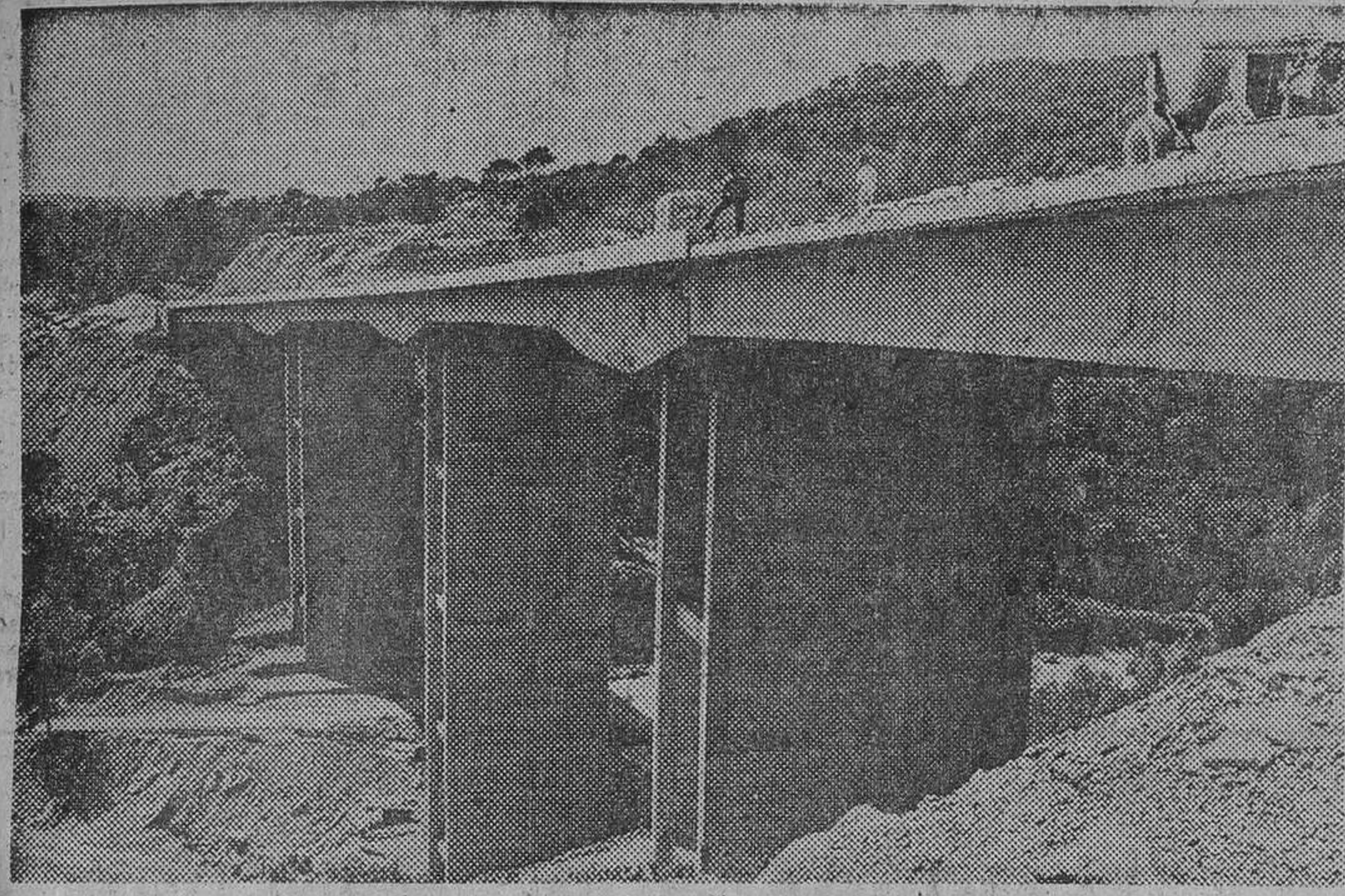
Uno de los dos viaductos gemelos de que constará el acceso al túnel de los Bruchs en plena obra de construcción.
