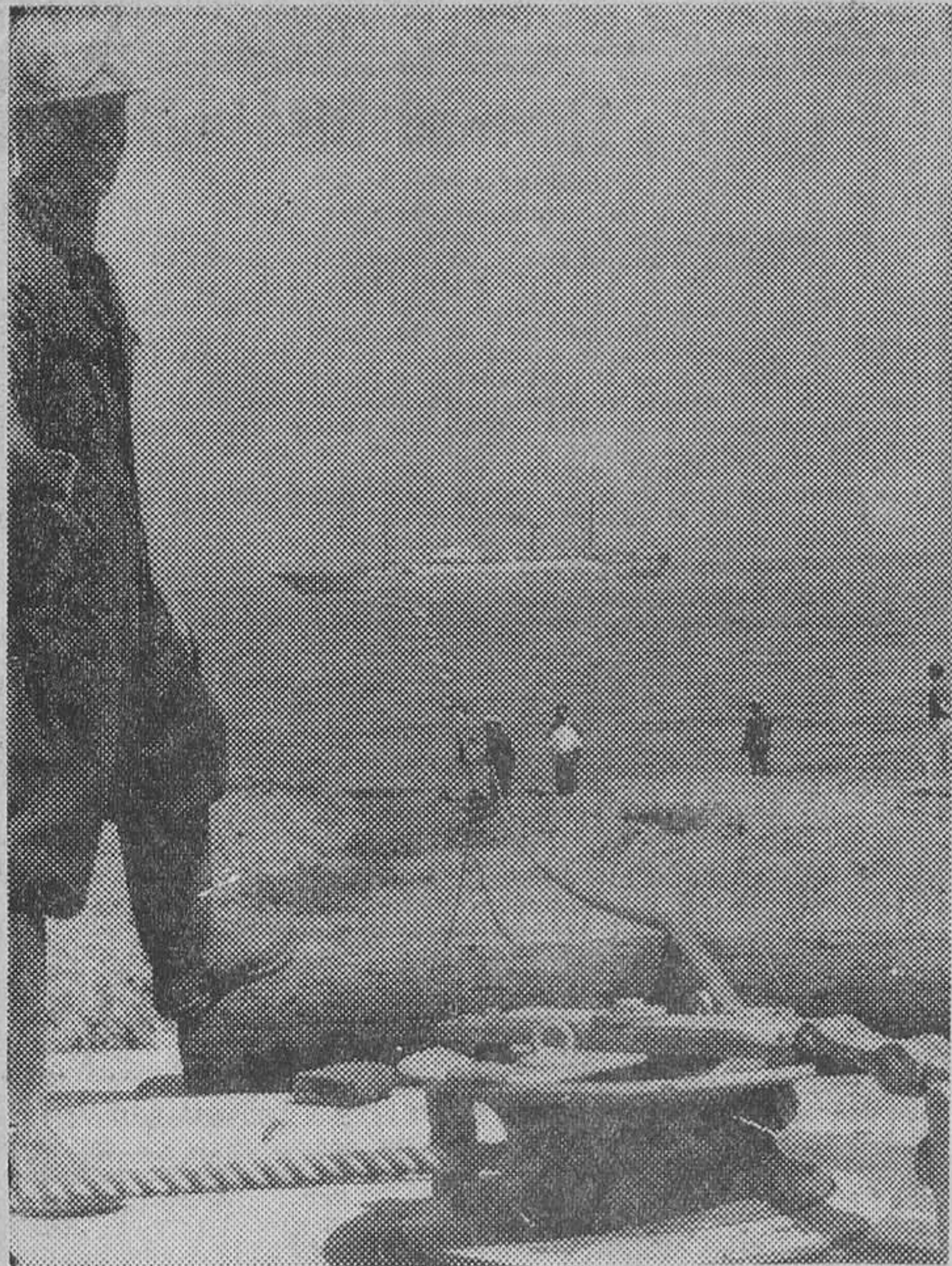
Momento de ser lanzado el cable axial que unirá telefónicamente Barcelona con Pisa, a través del cual podrán sostenerse 480 conferencias telefónicas simultáneas. (Foto Soterías)
