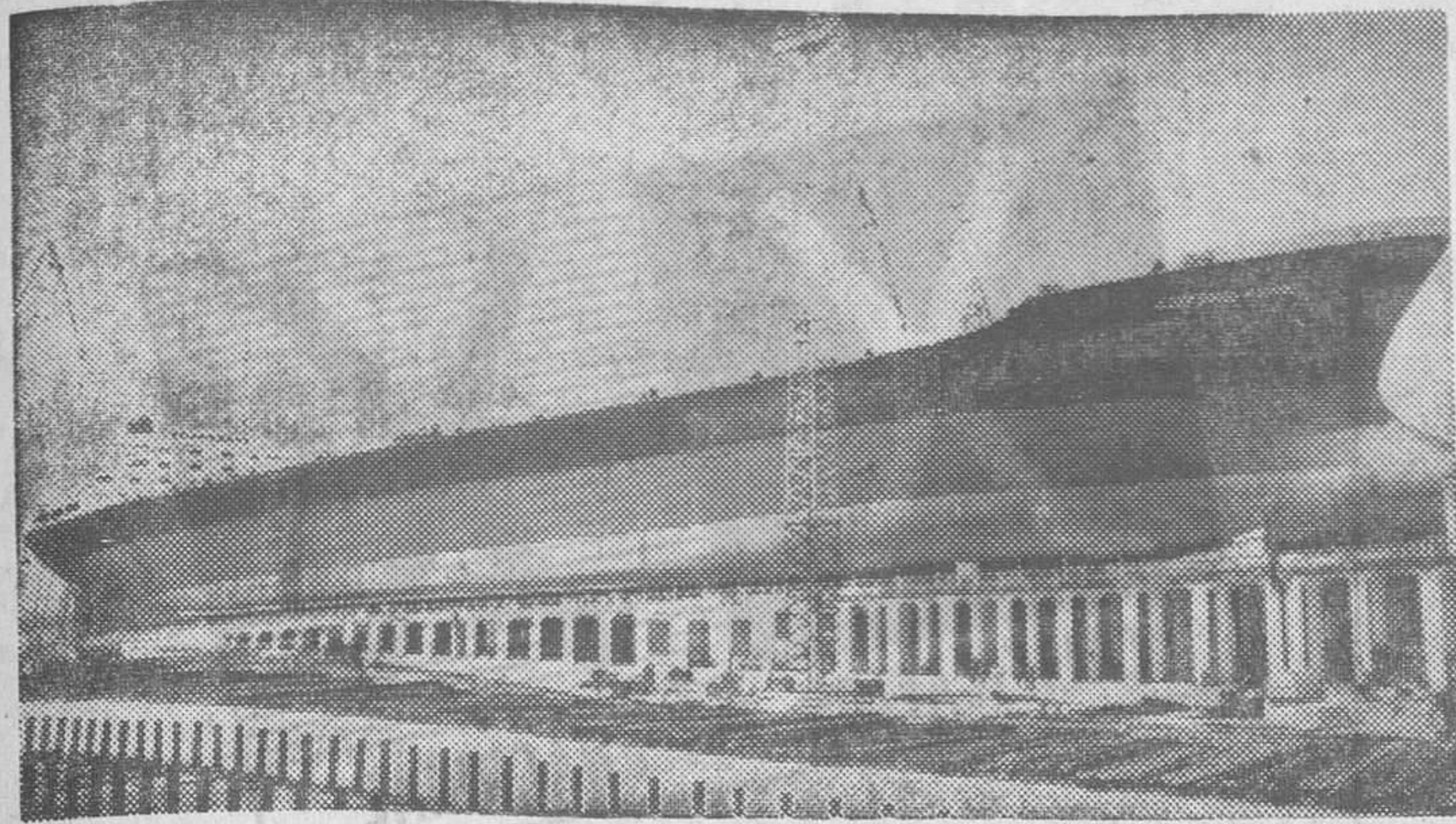
El Ferrol del Caudillo. — El petrolero «Idefonso Fierro», de 72.620 toneladas, que hoy será botado en los astilleros «Astano». Es el mayor que hasta la fecha se ha construido en España. (Foto Cifra)
