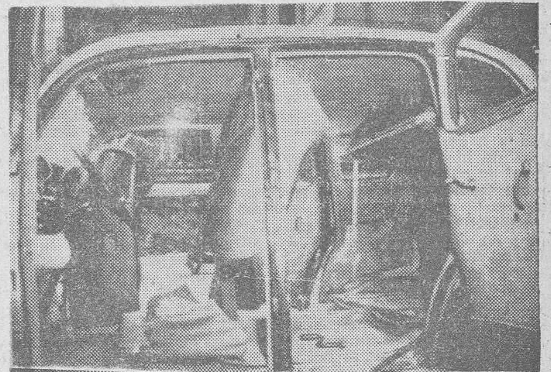
Interior del mismo coche, cuyos asientos, al girar por medio de especiales resortes, cubren sendas cavidades donde sus usuarios depositaban el contrabando. El compartimento disimulado por el asiento trasero es capaz para 300 kilogramos de mercancía
