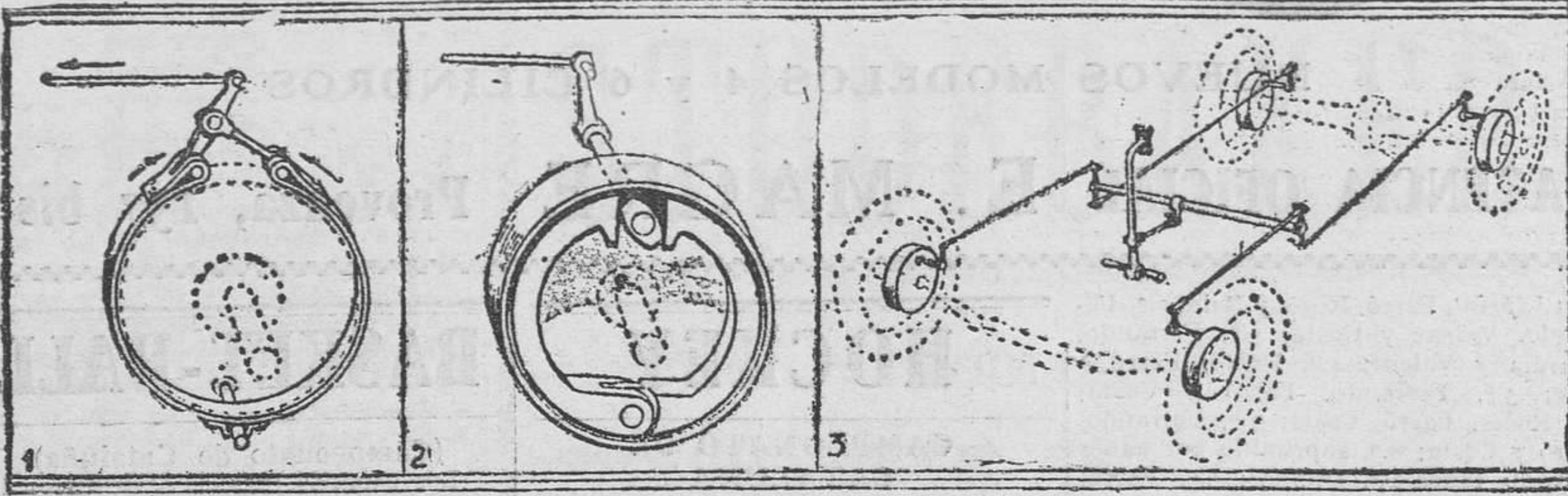
Fig. 1: Freno de banda de doble acción. Fig. 2: Un freno de expansión interna que consiste en dos zapatos pivotados en su parte inferior y obligados a entrar en contacto con el tambor por medio de una leva dispuesta en lo alto. Fig. 3: En el sistema de frenos sobre las cuatro ruedas, el eje cruzado aplica los cuatro juegos de zapatos cuando se pisa el pedal.
