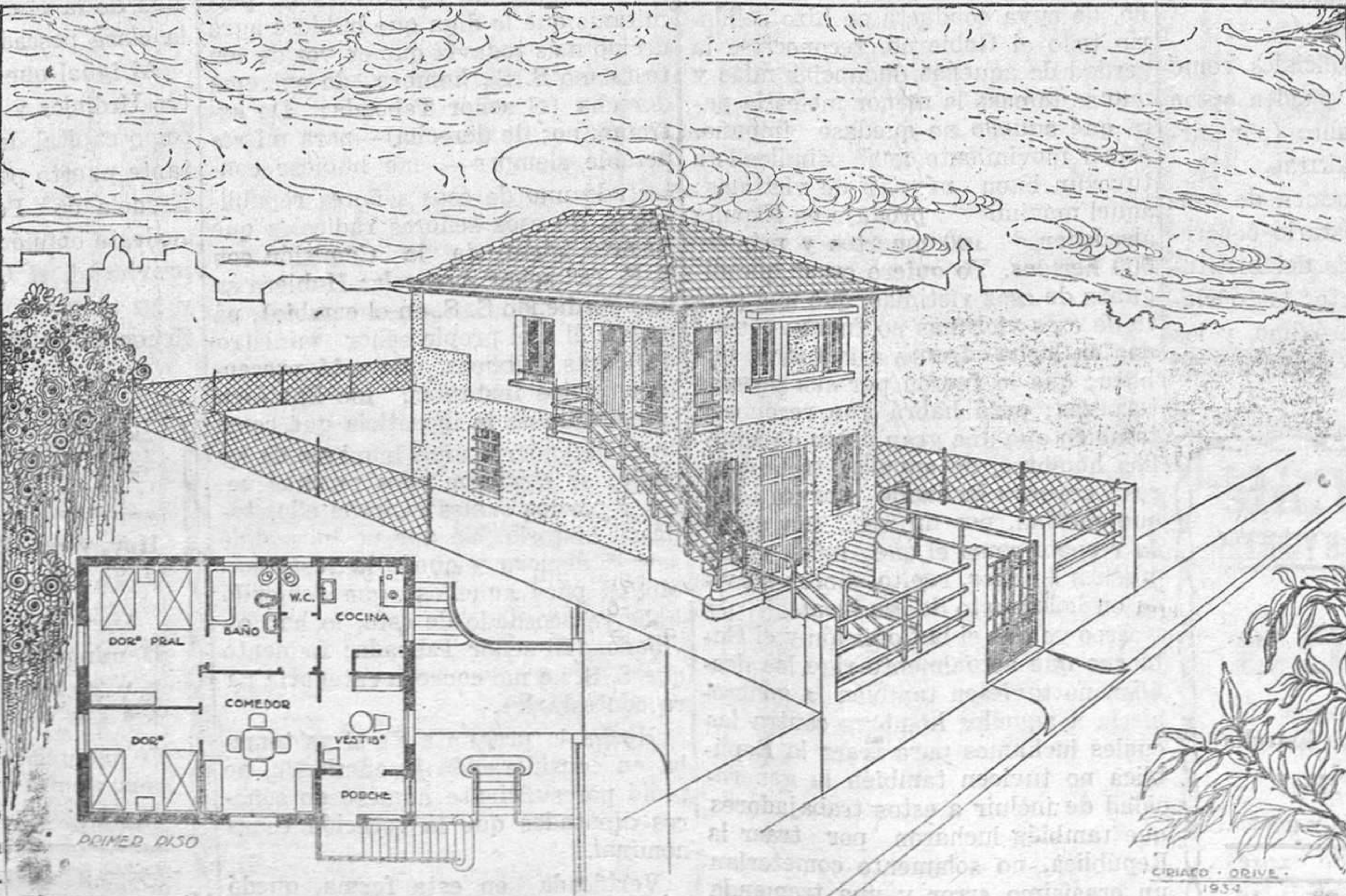
COOPERATIVA DE CASAS BARATAS "PABLO IGLESIAS". Proyecto de un chales proletario de Madrid. Dos plantas. Mide el solar 12 por 21,50 metros. Total, 258 metros cuadrados. Edificados, 89 y los 173 metros restantes dedicados a jardín. Presupuesto, 12.000 pesetas. Pagará al mes 54 pesetas. A los treinta años quedará amortizado su valor y habrá desaparecido el gasto mensual.
