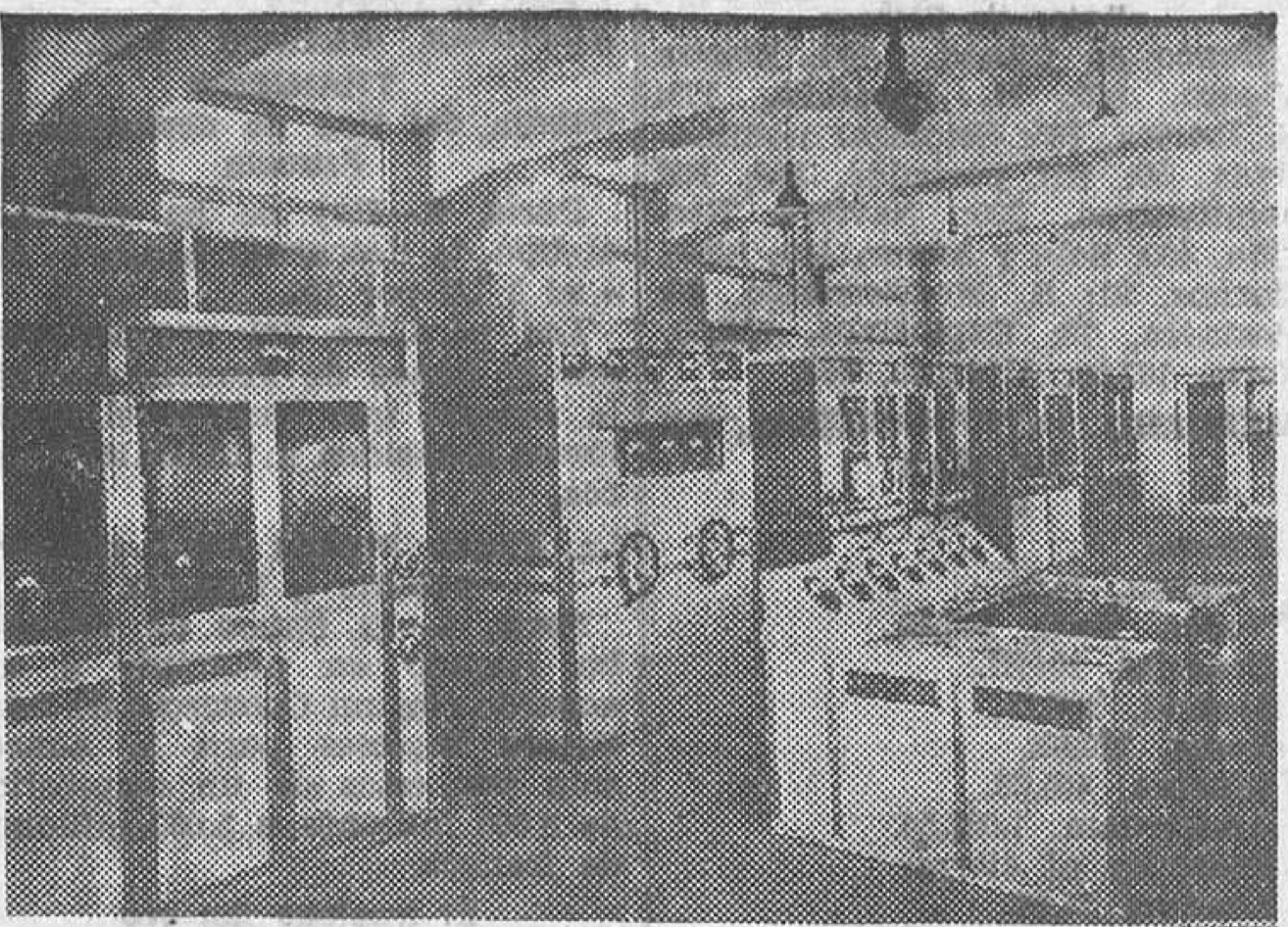
Vista interior de la emisora de 100 kilovatios de potencia, instalada por la Casa Marconi en Varsovia, que por la pureza de sus emisiones goza de prestigio técnico en Europa. Su antena mide 500 metros de altura
