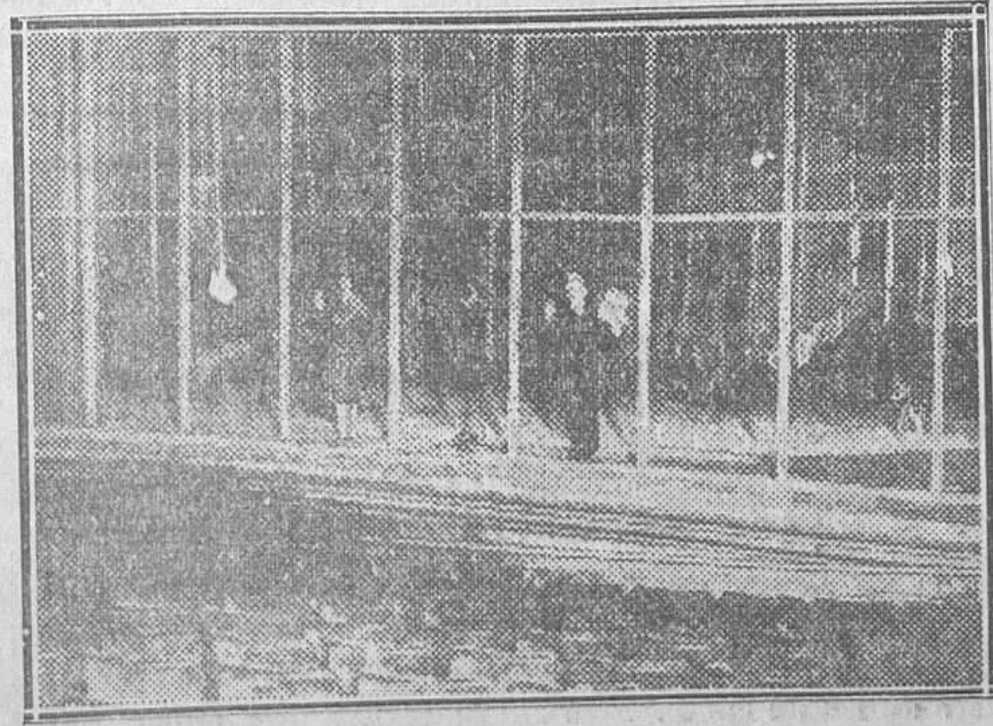
Estudio de una emisora americana, dividido en dos partes, separadas por una pared cristalina que sirve de pantalla al sonido. Los espectadores, cómodamente instalados en la sala, que es como la de un teatro, pueden presenciar la emisión sin que los ruidos que ellos producen lleguen al micrófono
