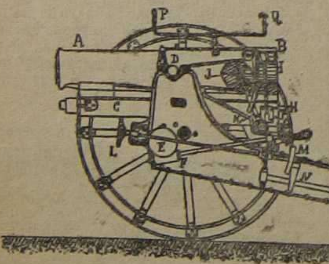
Figura 13.—Obús o mortero de campaña Krupp, de once centímetros y tiro rápido, adoptado por el ejército alemán
