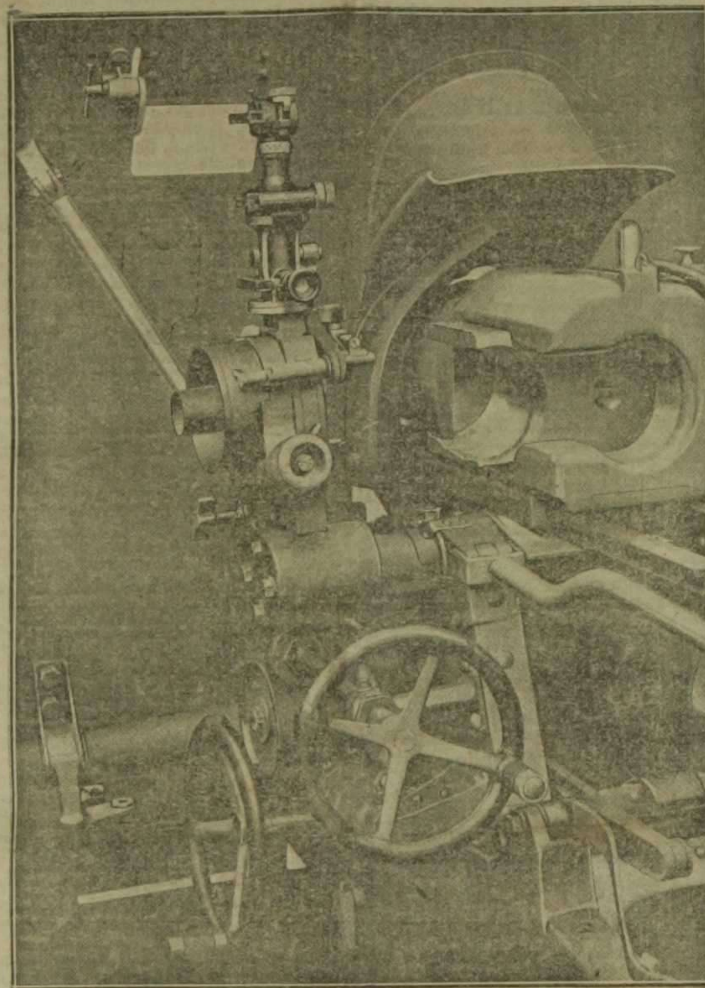
Telómetro de la casa Goerz, que descubre un amplio panorama, aplicado sobre un mortero de las fábricas de Krupp, en Essen-Ruhr (Alemania)
