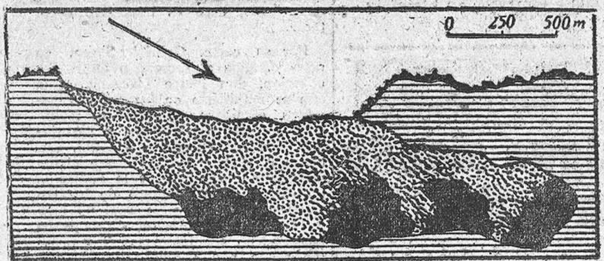
Esquema, según Buerger, de los trozos en que se fragmentó el bólido caído sobre Arizona hace cincuenta mil años.
