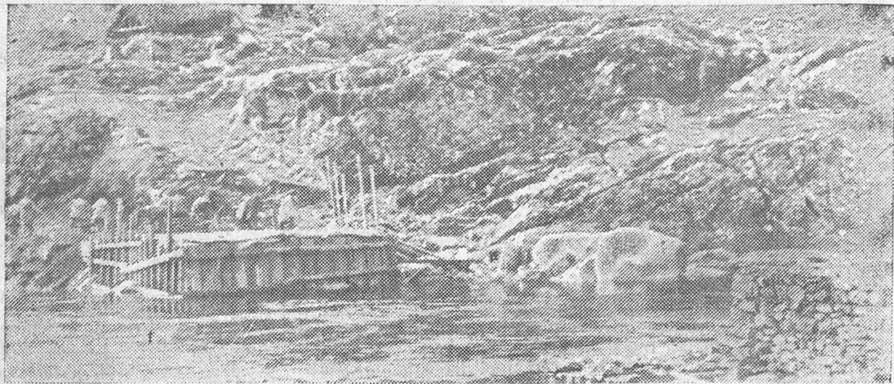
El puente de hierro que se está construyendo se espera que entre en servicio mañana. Los cimientos ya están, como puede verse en la presente «foto». Ahora sólo falta tender el armazón metálico.
