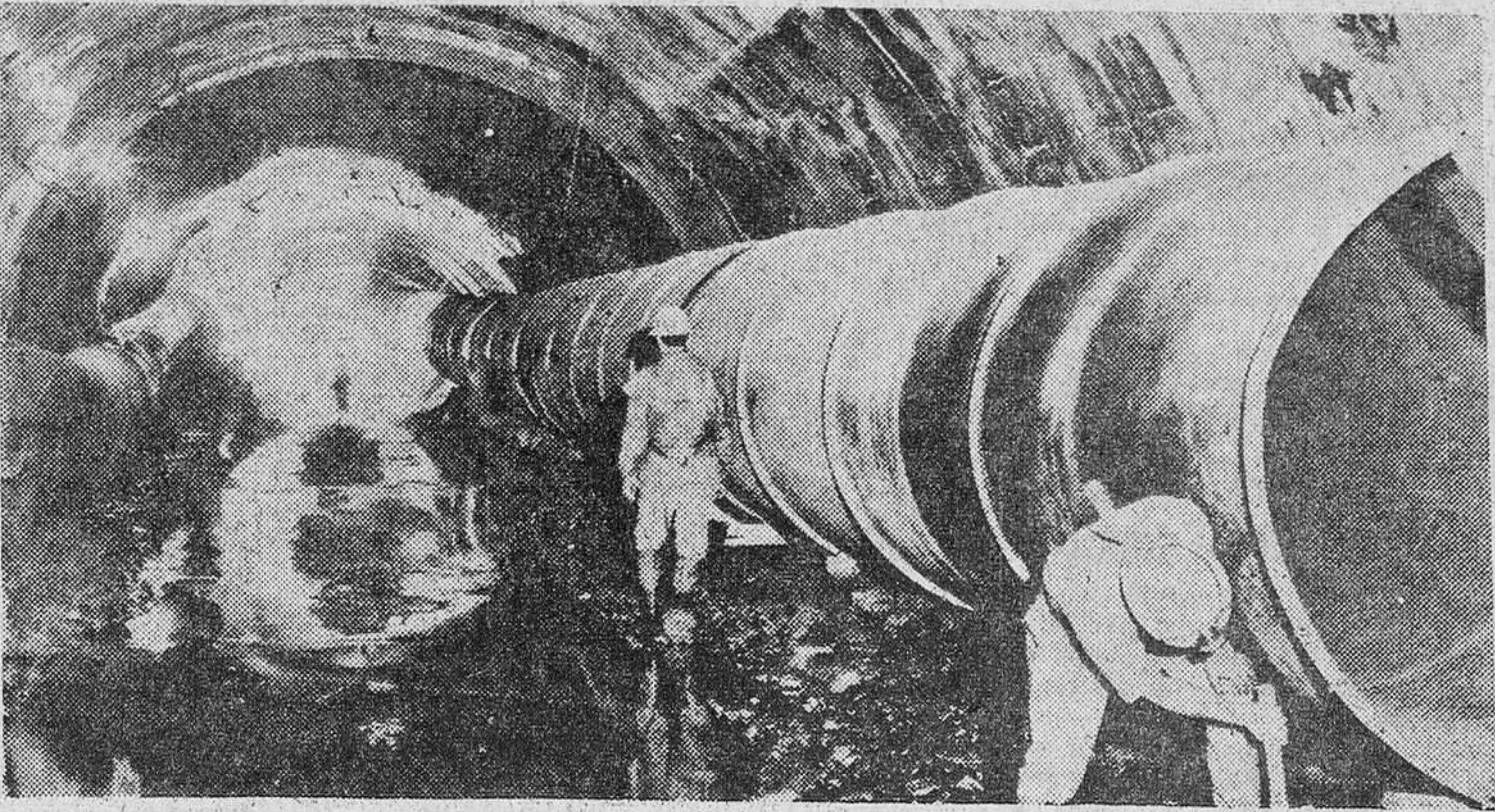
Grandes obstáculos estorbaban las obras, en la parte italiana, por la cantidad de esquistos desprendidos y emanaciones de agua. La gran tubería es la de conducción de aire viciado.
