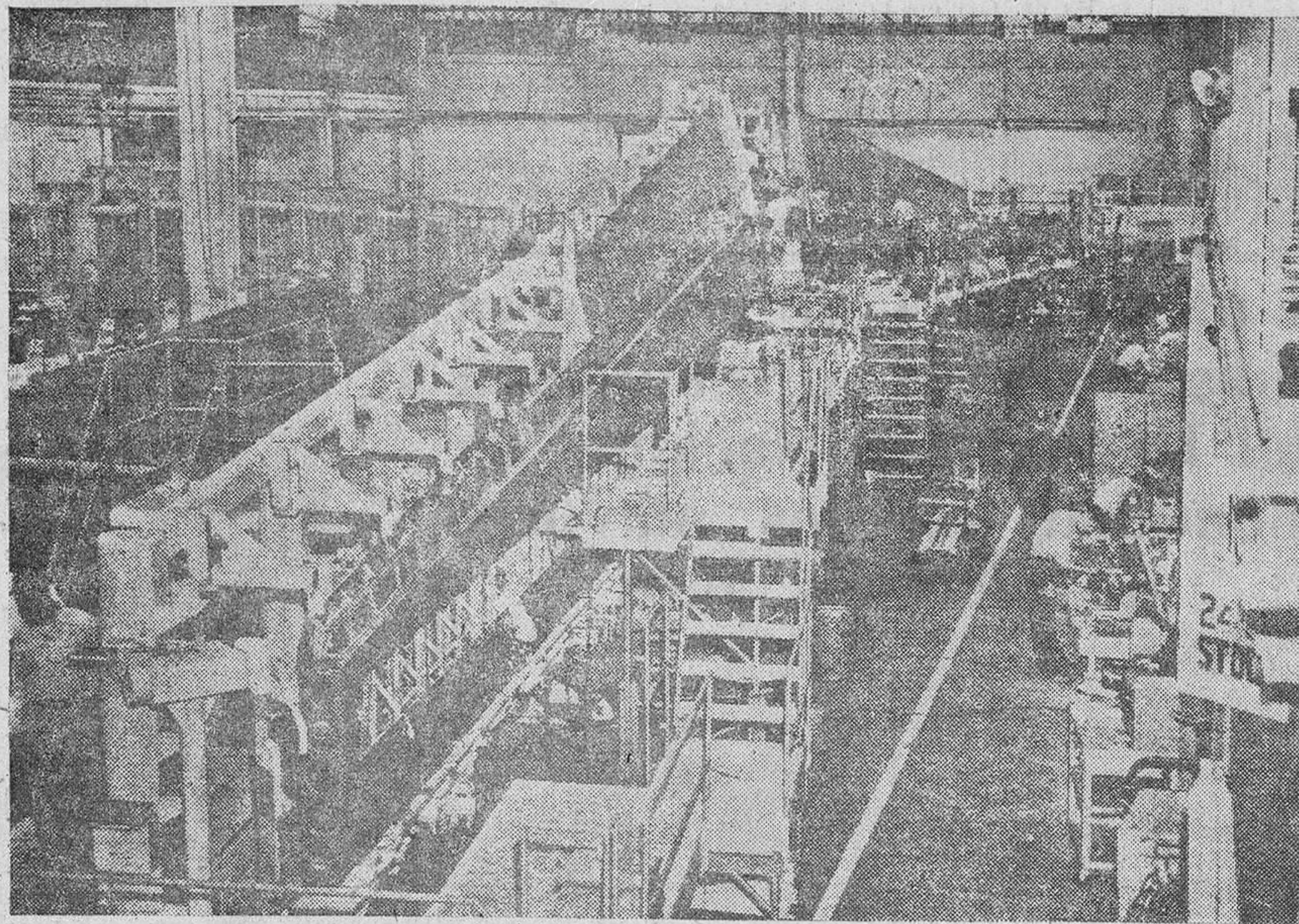
Estos talleres se ocupan en la construcción del ala más larga para aviones de uso civil. Las nuevas alas (150 pies de longitud) proporcionarán al avión una autonomía de más de once mil kilómetros.
