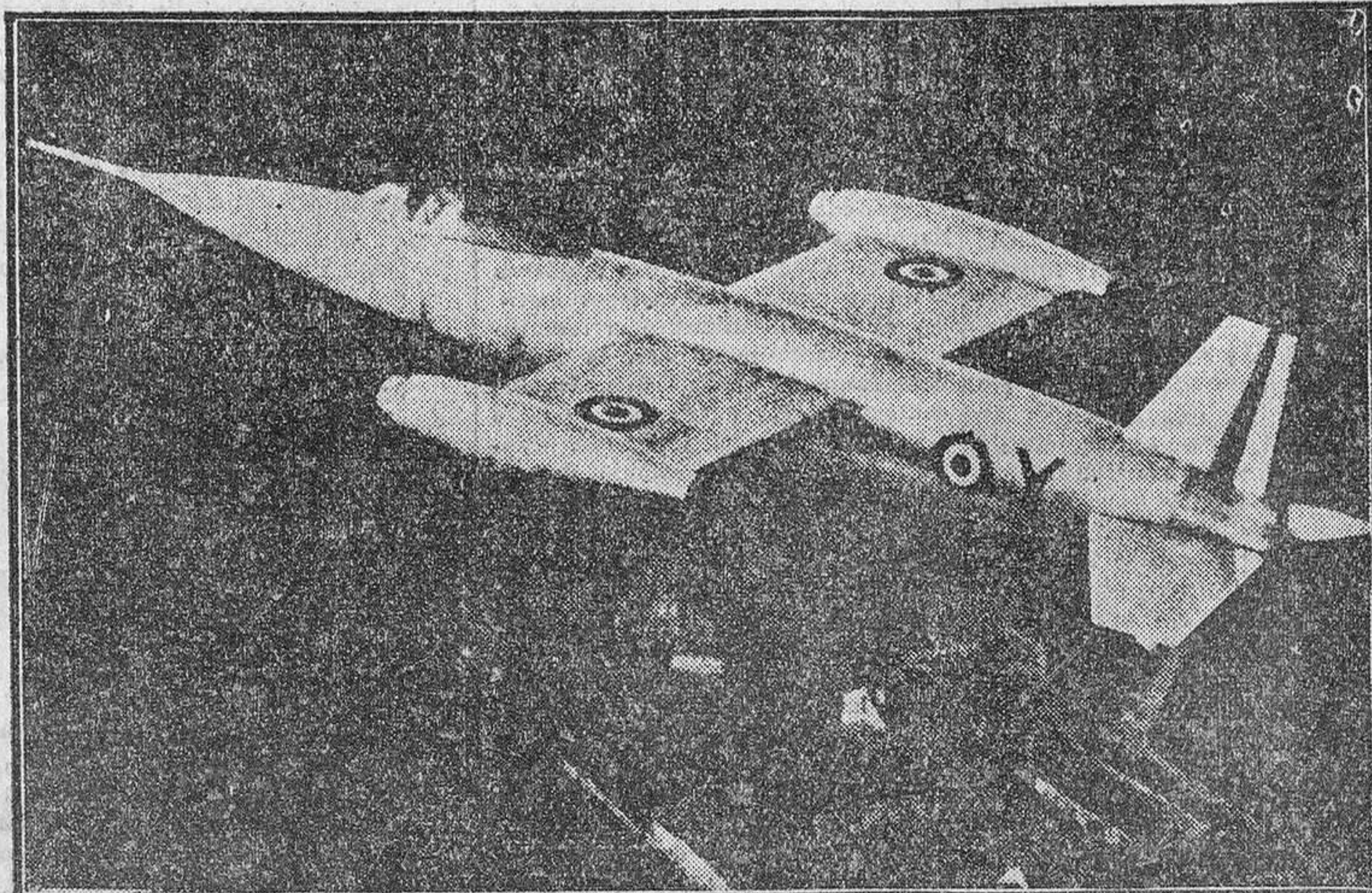
Este aparato experimental, el "Tritón" que, como es natural, no será presentado en ningún salón, es la esperanza de la aviación francesa. Se espera que permitirá realizar desplazamientos supersónicos a un precio quince veces más económico que los actuales. Su carburante será ácido nítrico, y la velocidad calculada, mil ochocientos cincuenta kilómetros por hora. Como especial dispositivo de seguridad, la cabina podrá ser proyectada automáticamente al espacio como paracaídas, en caso de accidente.
