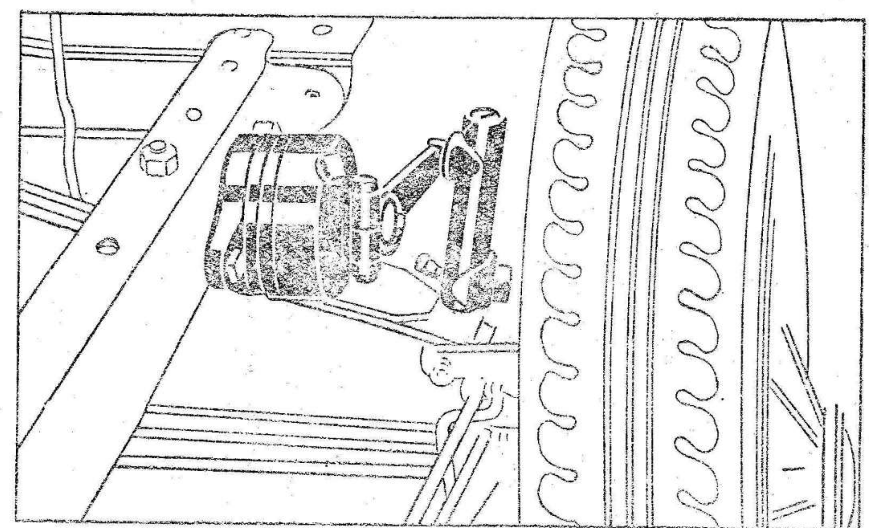
Detalle del amortiguador
