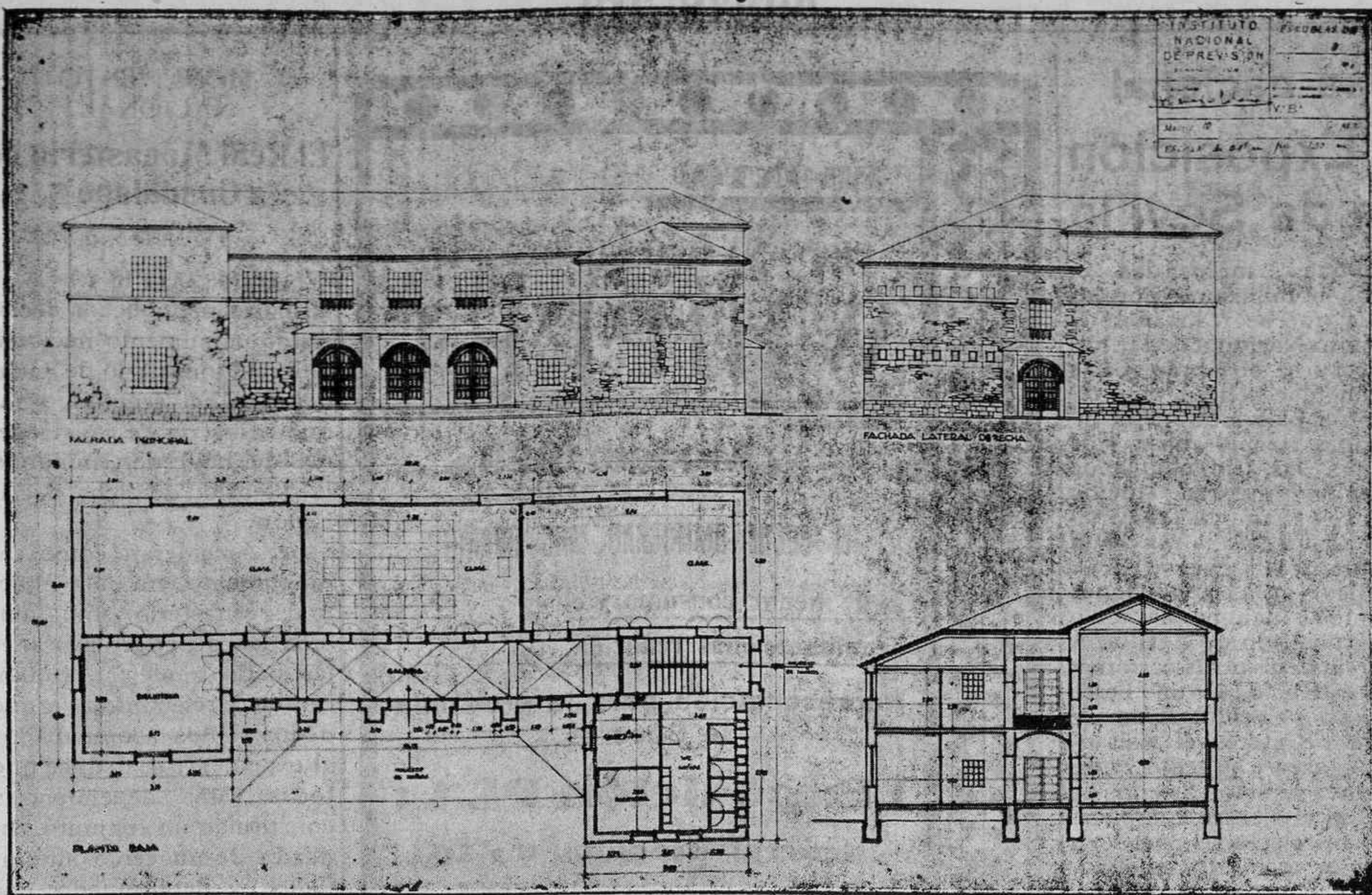
Planos de las escuelas de Losar de la Vera, cuya construcción, en subasta celebrada ayer, fué adjudicada por la cantidad de 119.899 pesetas al contratista de obras públicas, de Plasencia, don José Rodas Calderón
