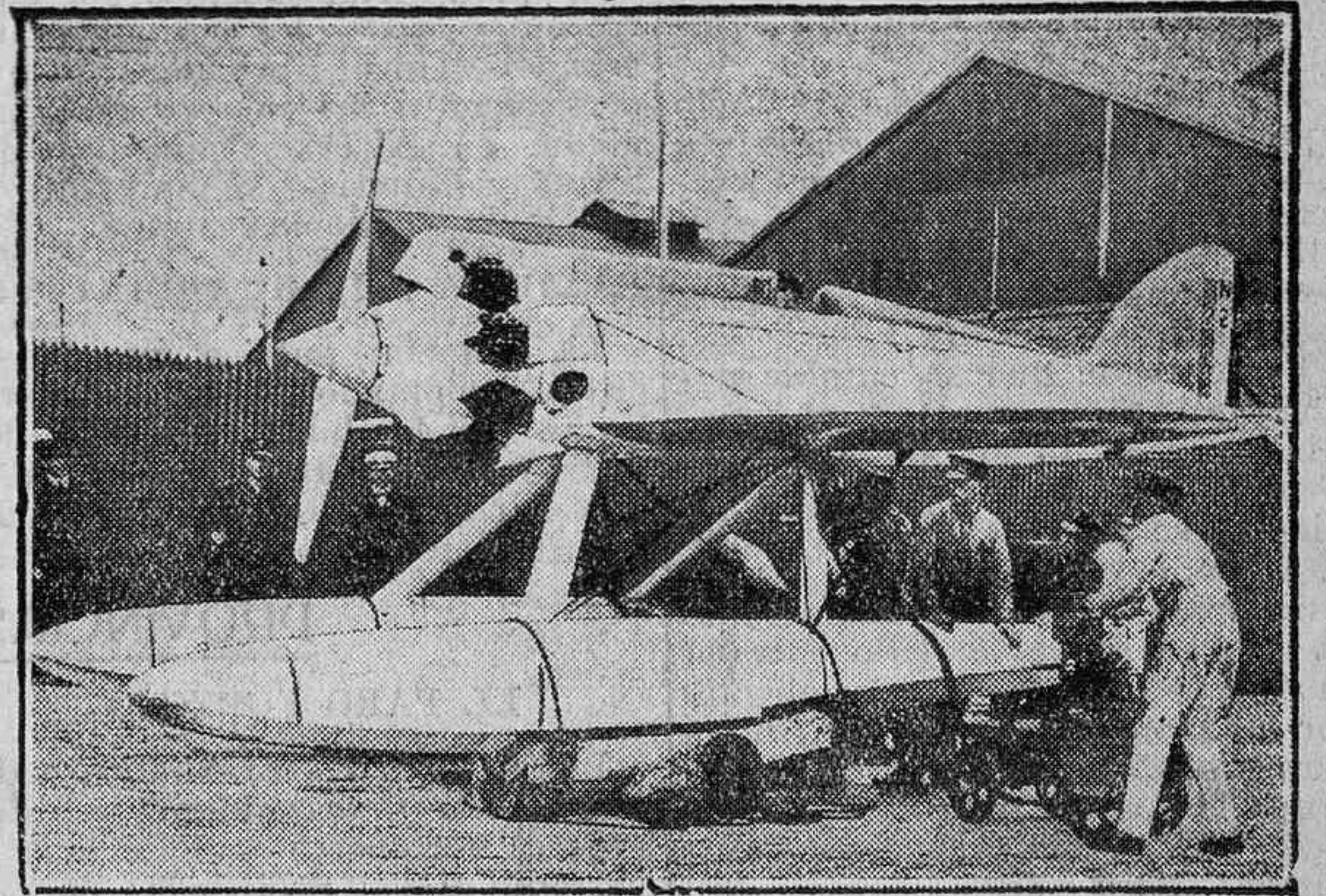
Inglaterra ha construido, en medio del mayor secreto, un hidro-aeroplano (nuestra foto) de gran velocidad, con el cual piensa ganar la copa «Schneider», de velocidad, en la competición internacional que se celebrará en Venecia en septiembre próximo.
