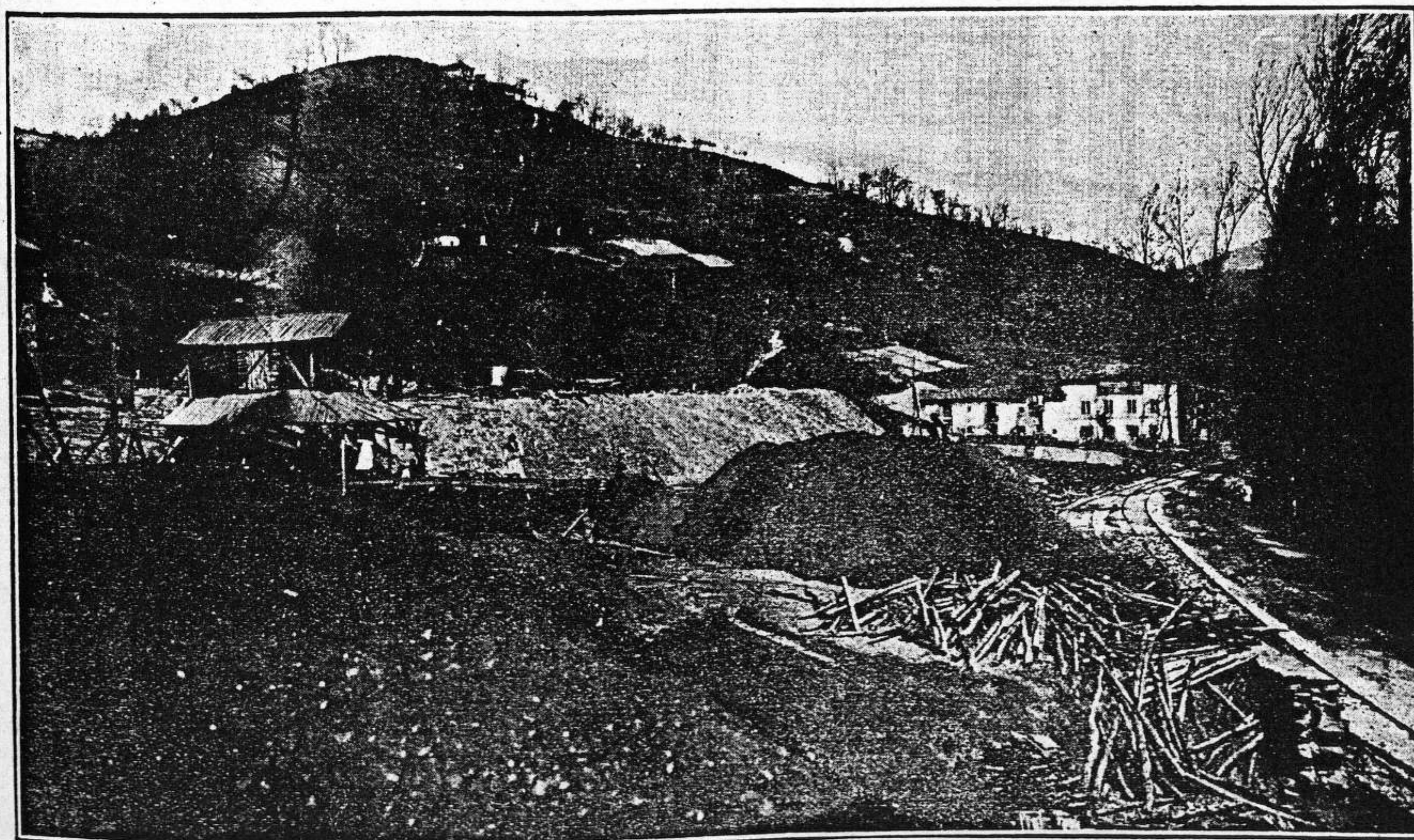
LANGREO.—Mina "El Campanal" con cargadero sobre el ferrocarril
