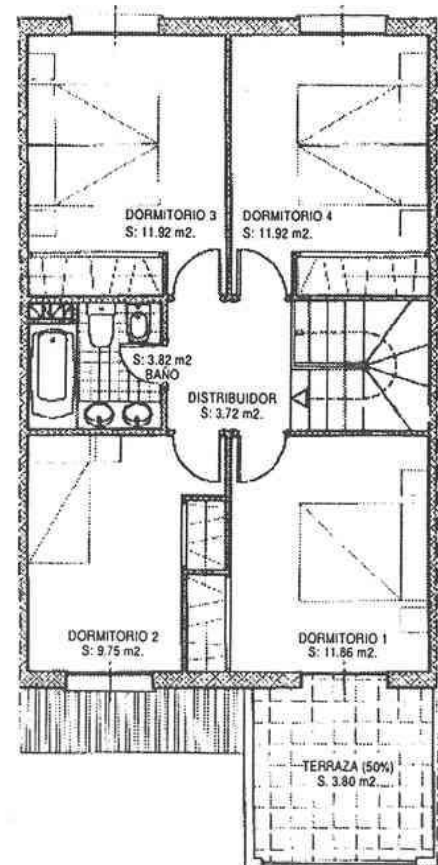
PLANTA ALTA
