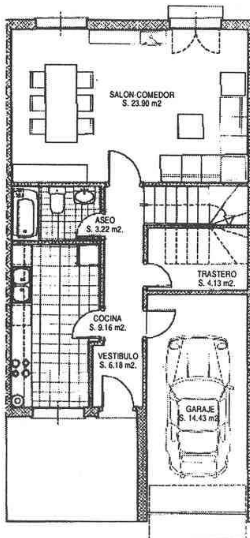
PLANTA BAJA
