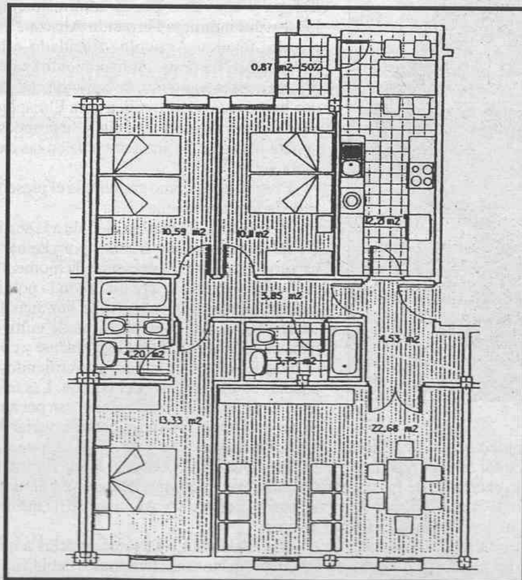
Plano piso 3 dormitorios
