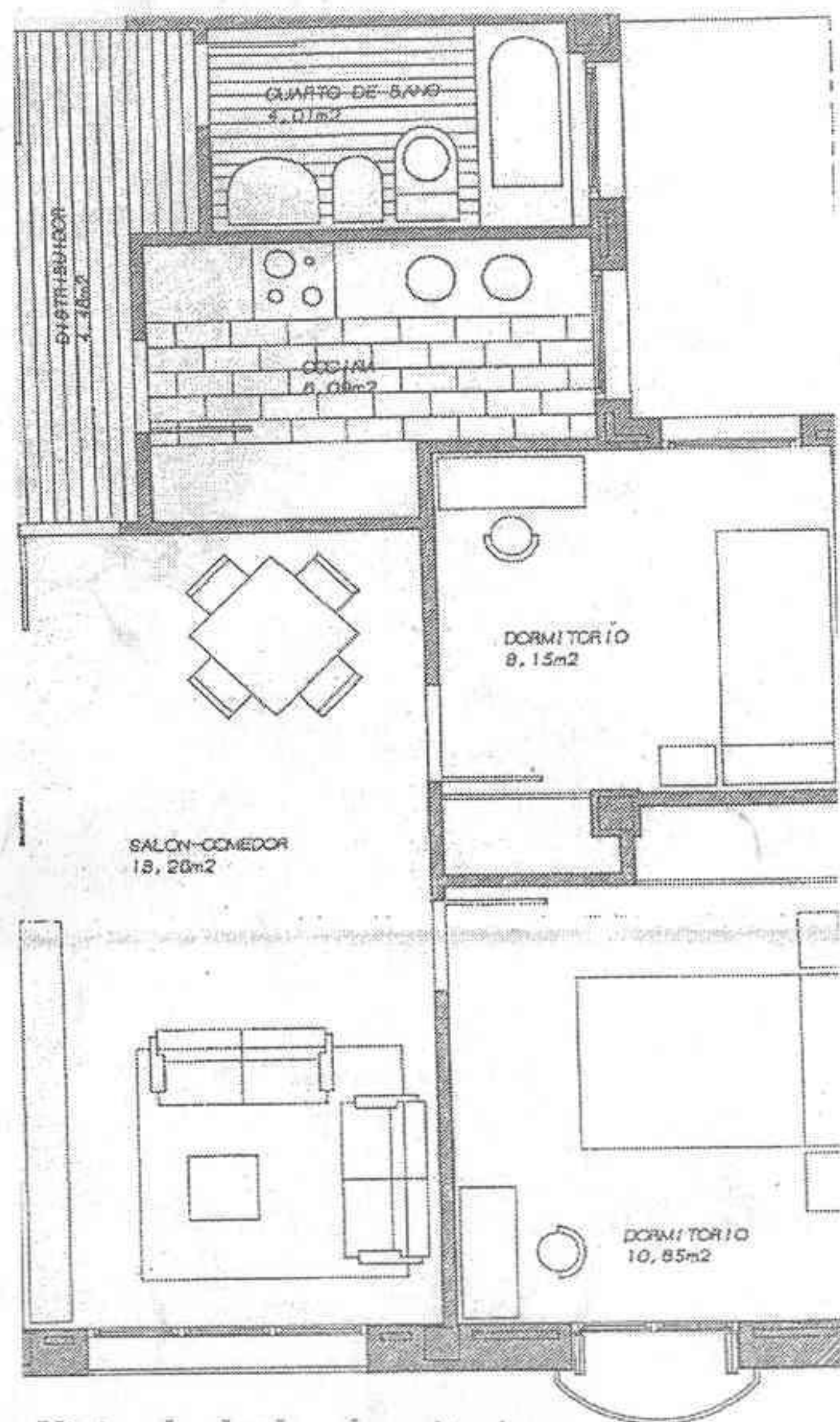
Vivienda de dos dormitorios Sup. construida 69,01 m 2
