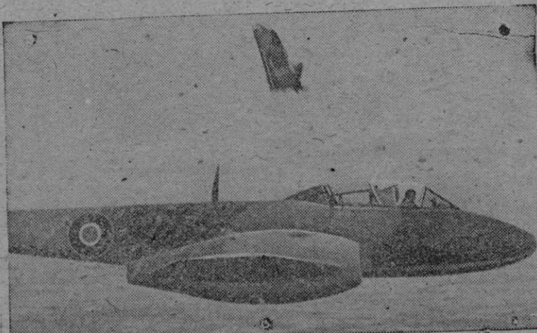
En todos los aviones modernos de la R.A.F. se han montado asientos de expulsión para los pilotos. En la fotografía puede verse uno de ellos en el aire, después de abandonar el aparato en unas pruebas celebradas recientemente
