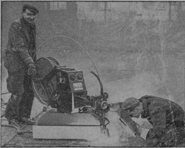
El aparato soldador "Fusarc" empleado en la soldadura de planchas de un buque en construcción en unos astilleros de Belfast
