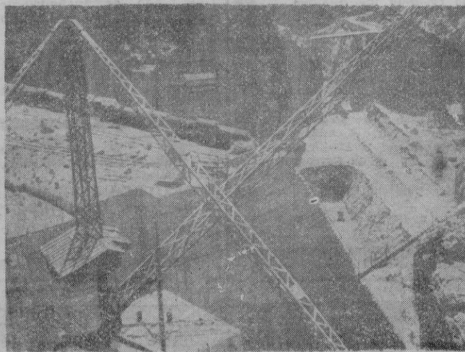
Una vista de las obras que actualmente se realizan en el Pantano del Generalísimo, que embalsará 60 millones de metros cúbicos de agua y que se calcula será terminado a este año 1949. (Foto «Cifra Gráfica»)
