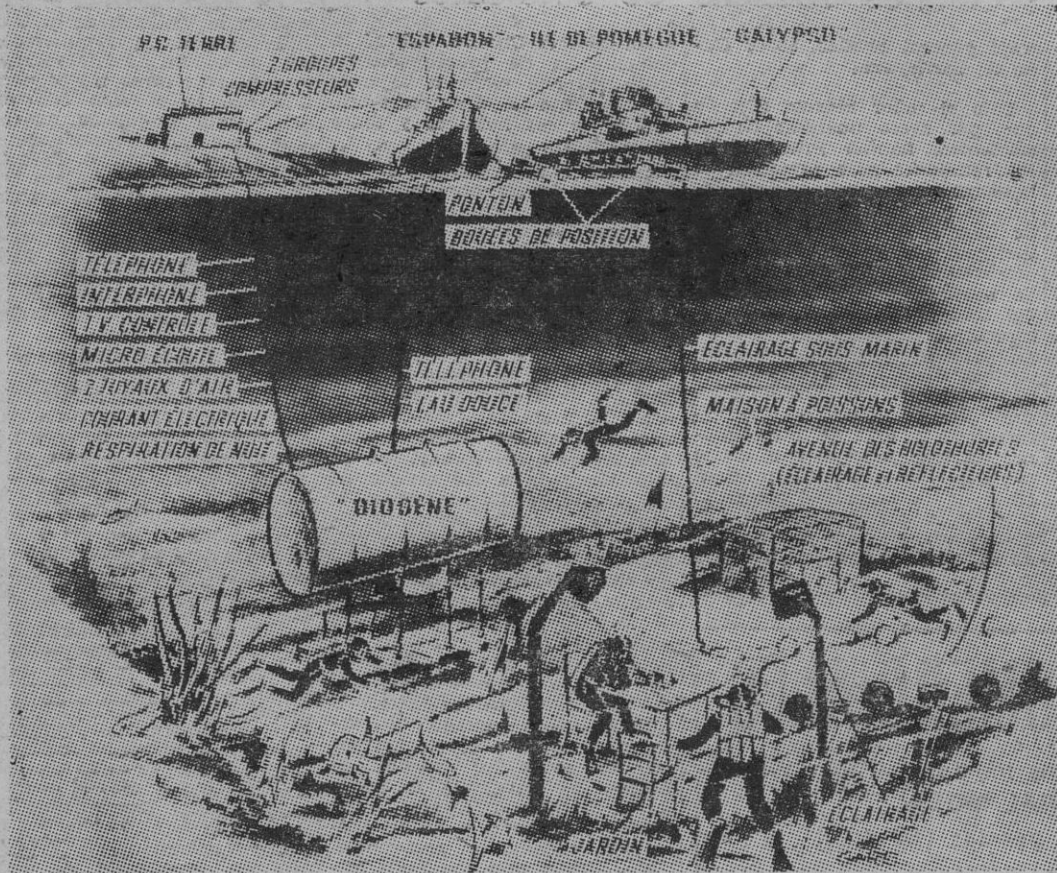
Representación gráfica de la finca submarina, con su jardín, avenida de las Holturias, jaula para los peces y conexiones con tierra y con los buques del comandante Cousteau. (Foto Fiel.)
