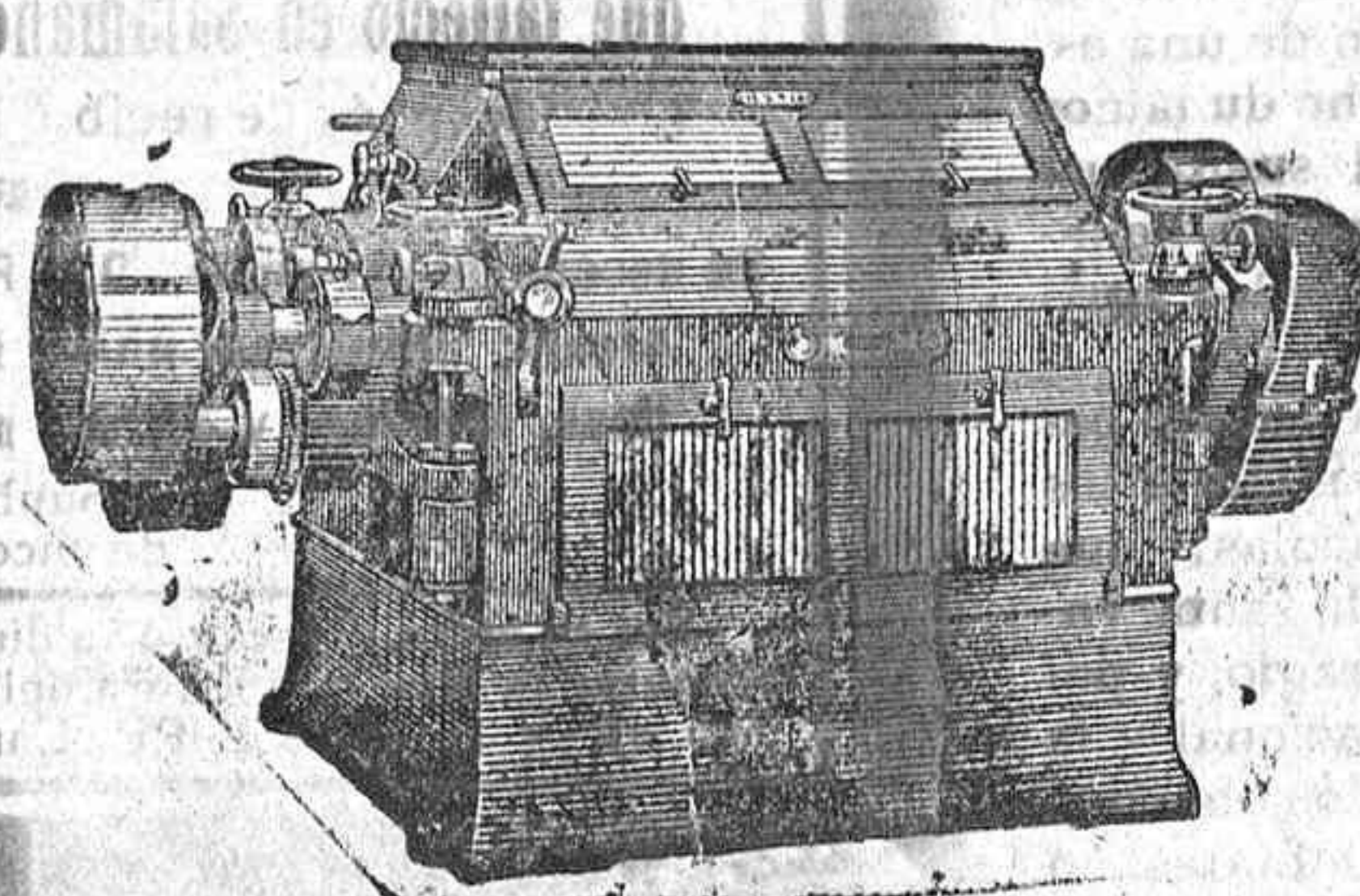
Molino modelo DD de cuatro cilindros. Privilegio BÜHLER
