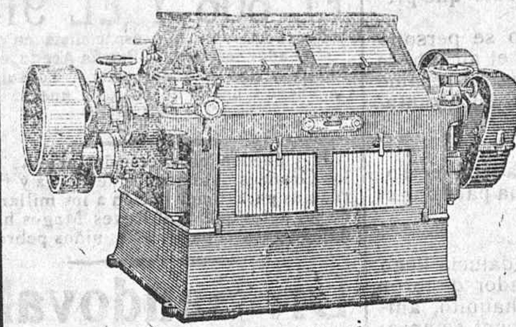
Molino modelo DD de cuatro cilindros. Privilegio BÜHLER
