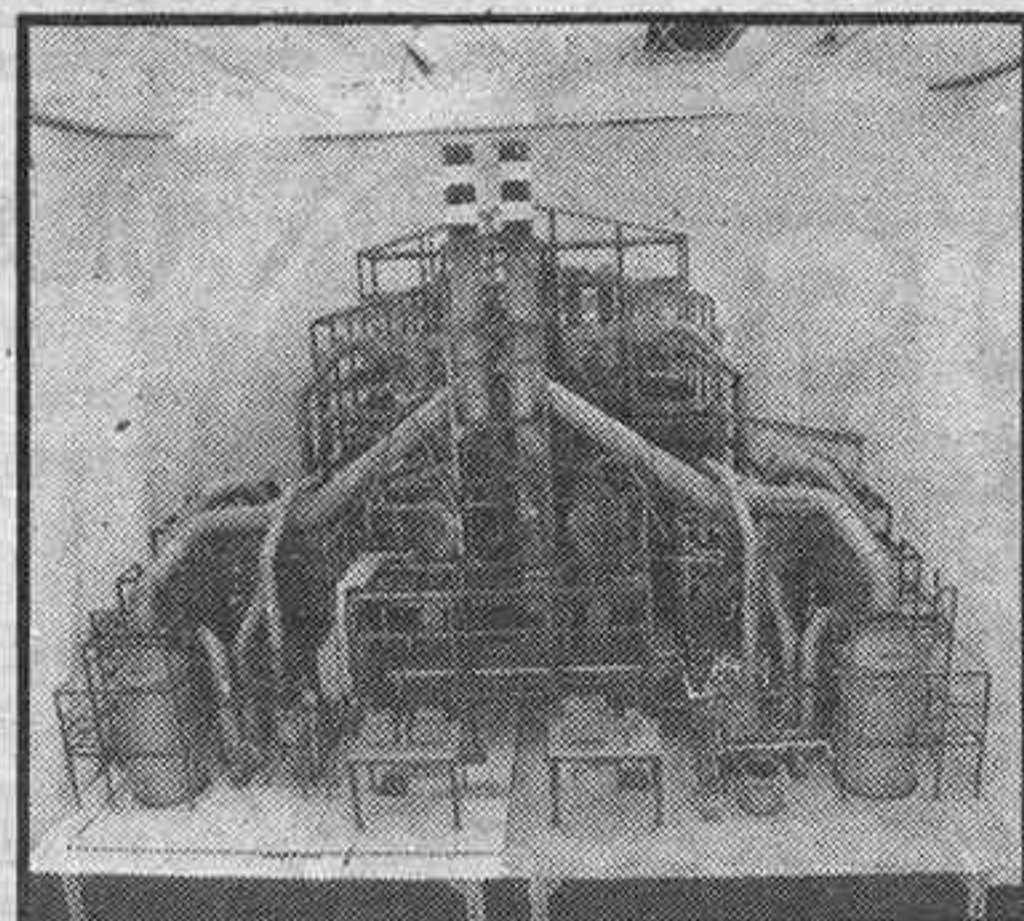
Maqueta de las unidades de proceso de granulación y sulfato amónico, para Filipinas. El valor material solamente de la maqueta es de cuarenta millones de pesetas
