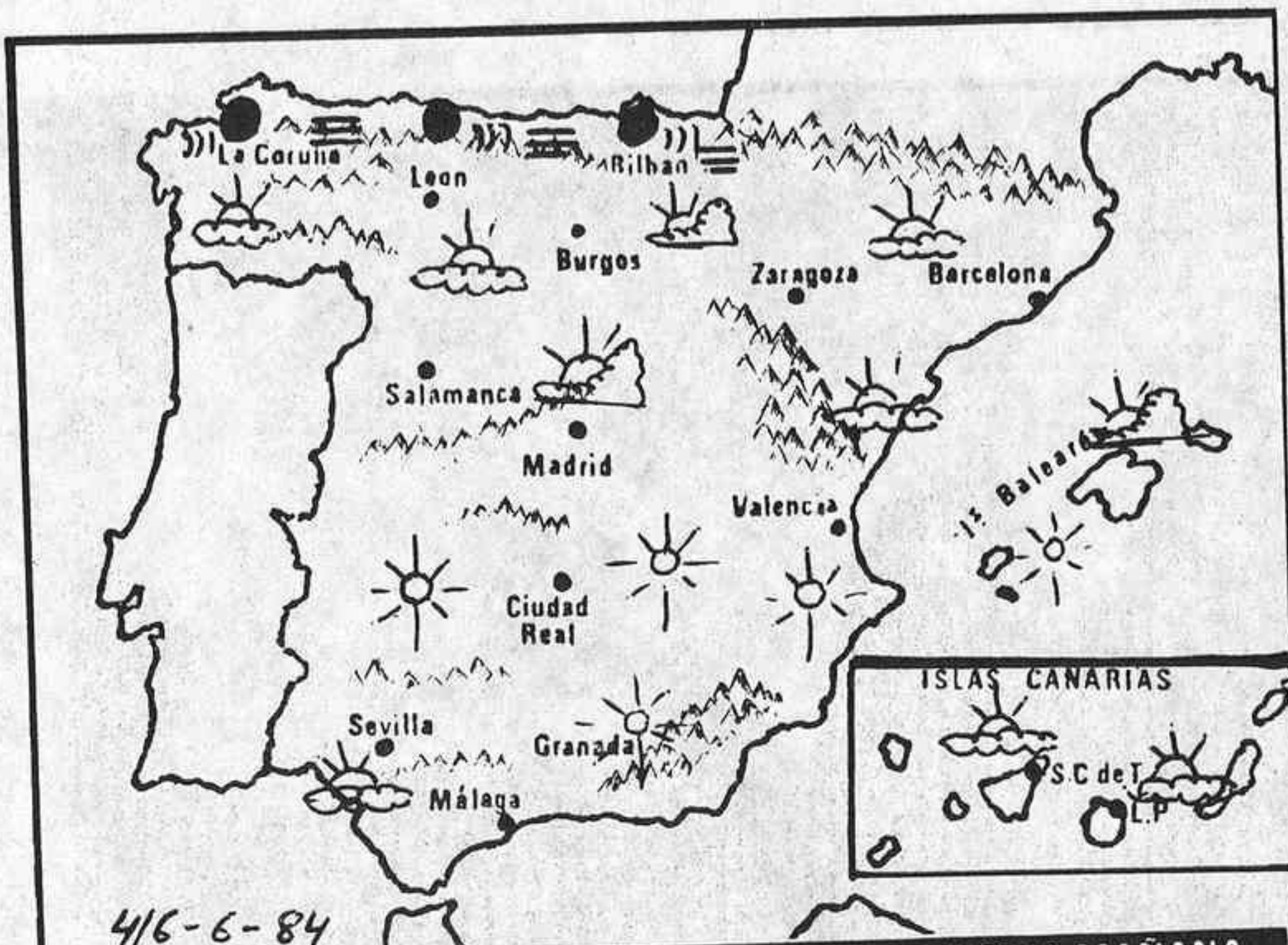
ESTADO DEL CIELO Y METEOROS PROBABLES DE HOY A MAÑANA
