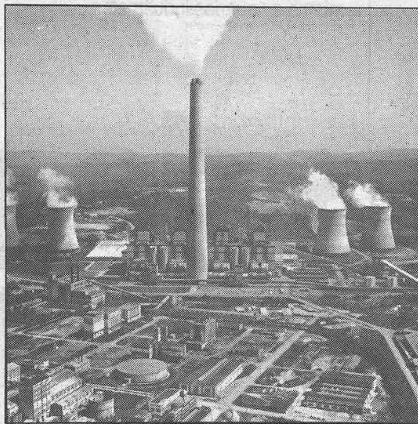
Central térmica Puentes de García Rodríguez (La Coruña). Cuatro equipos de 350 MW
