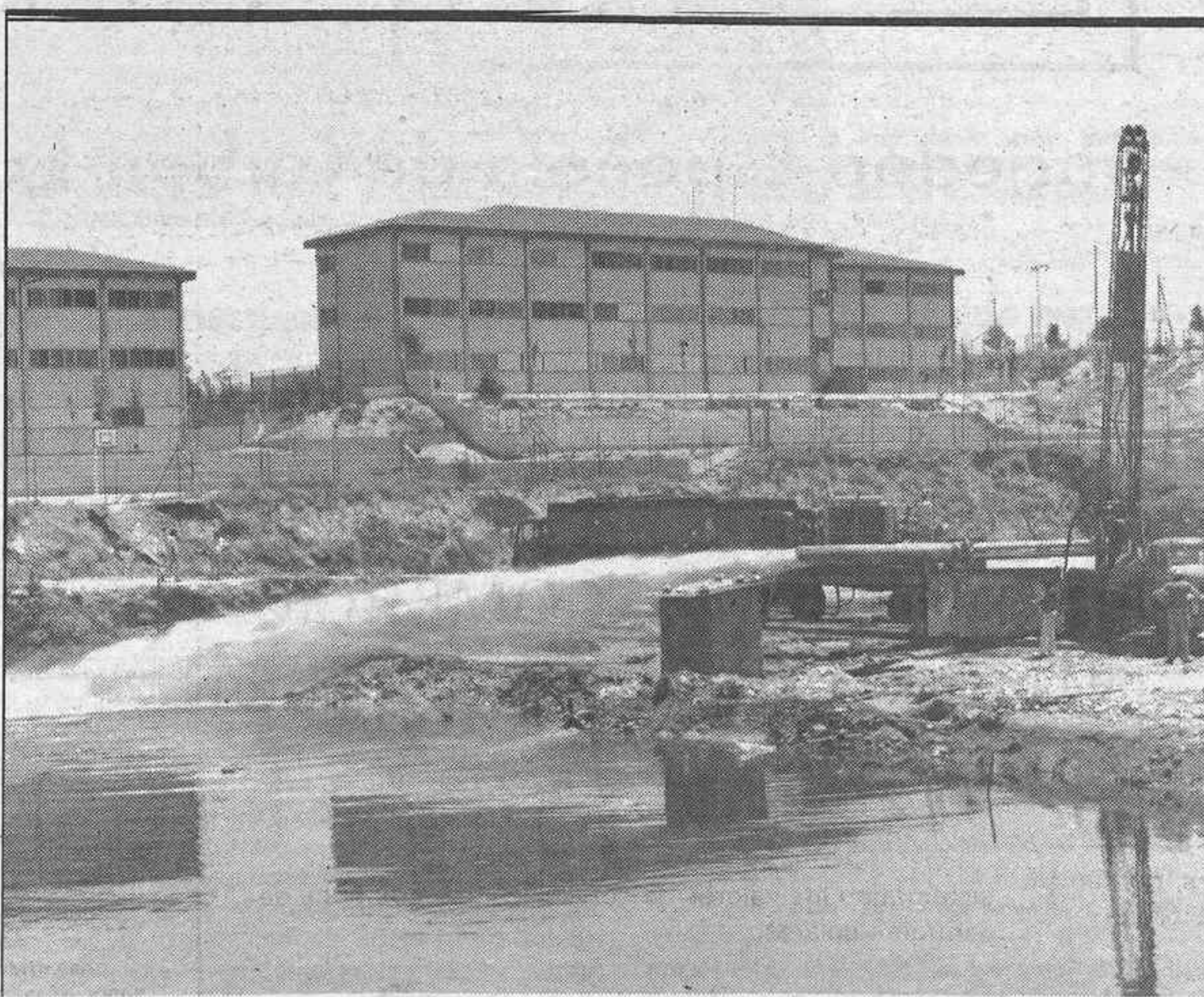
En el Centro Asistencial de Mondragón (Guipúzcoa) se ha establecido para climatización de la zona de quirófanos un dispositivo de dos unidades de bomba de calor, con una potencia eléctrica de 16,5 kilovatios, con un consumo anual de 38.504 kilovatios hora. La energía aportada al conjunto por la bomba de calor es de 143.233 kilovatios hora al año, con un ahorro de costes de energía en el mismo período de 336.000 pesetas y un ahorro de gasóleo de 18.300 litros, todo lo cual permite amortizar la instalación en tan sólo dos años. En la fotografía, enmarcada en el bello paisaje de la localidad guipuzcoana, una visión parcial de estas interesantes instalaciones
