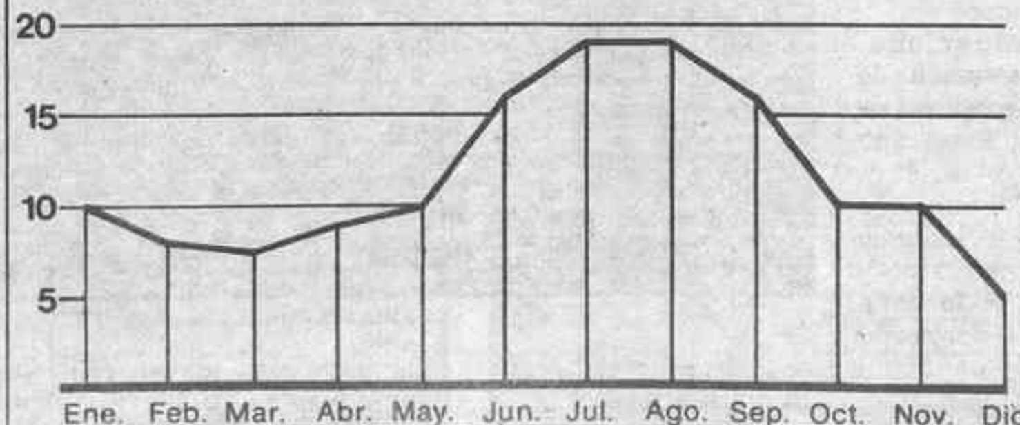
El agua de refrigeración que se devuelve al Tajo podría elevarse en el caso más desfavorable (caudal mínimo) en un máximo de tres grados. Debemos tener en cuenta que las diferencias de temperaturas naturales pueden llegar a alcanzar variaciones de hasta 15° grados
