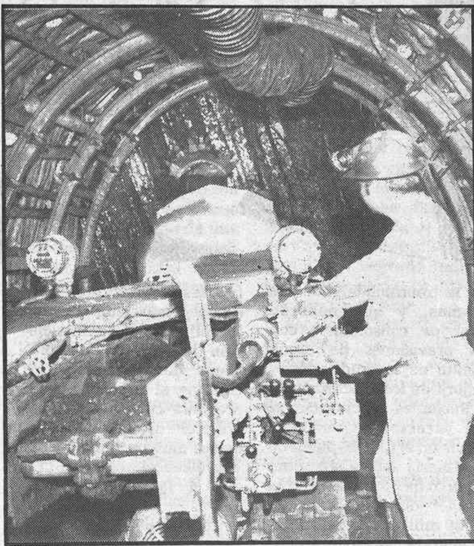
Avance mecanizado en una galería de carbón
