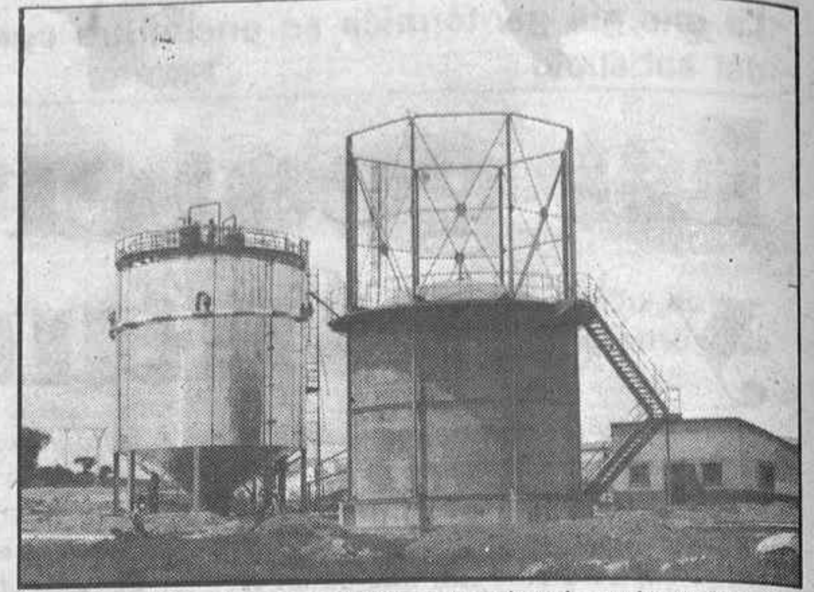
Digestor 500 m 3 - Sistema DAC - para purines de porcino en Mérida
