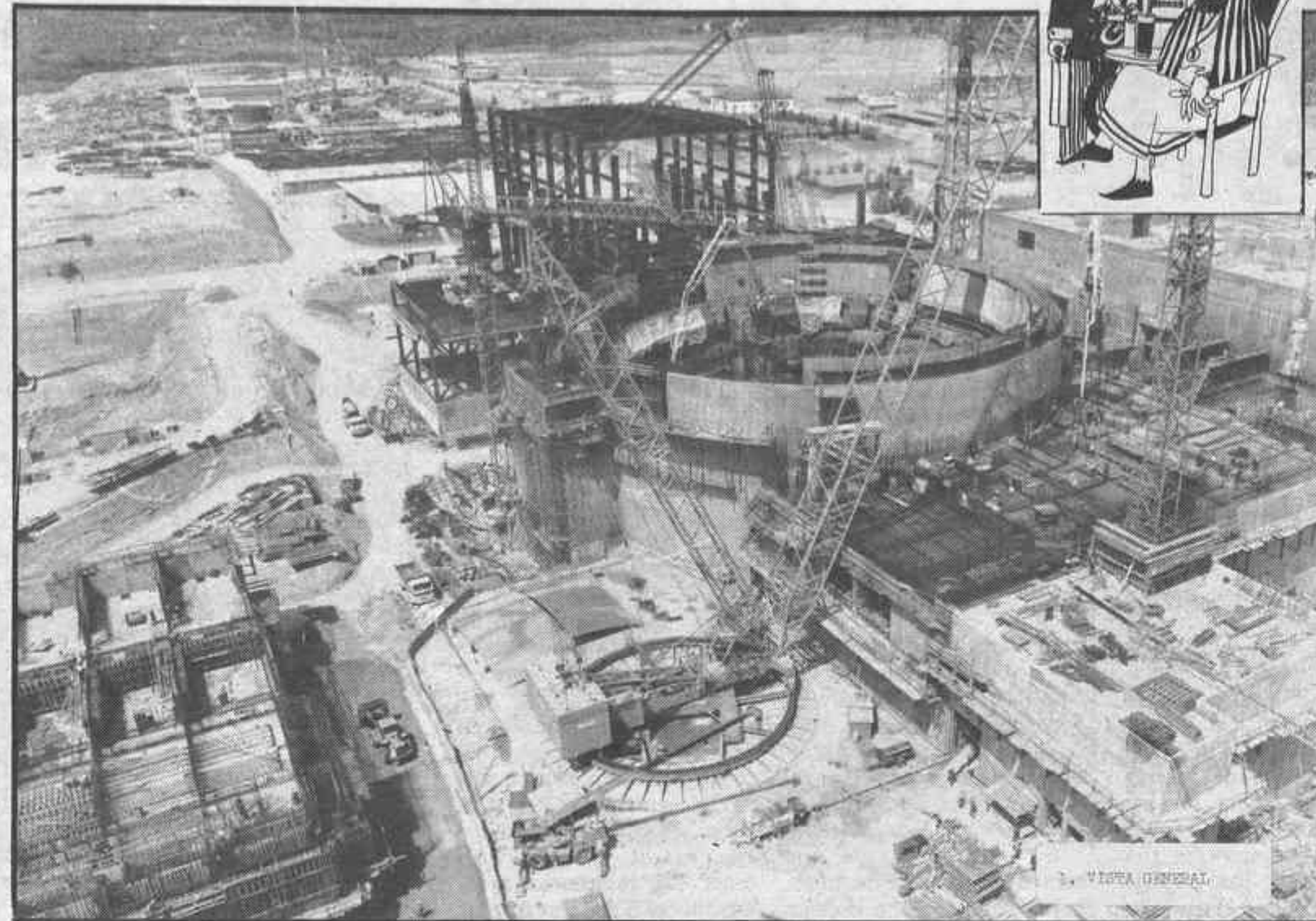
Panorámica de las obras de la central de Trillo en la actualidad
