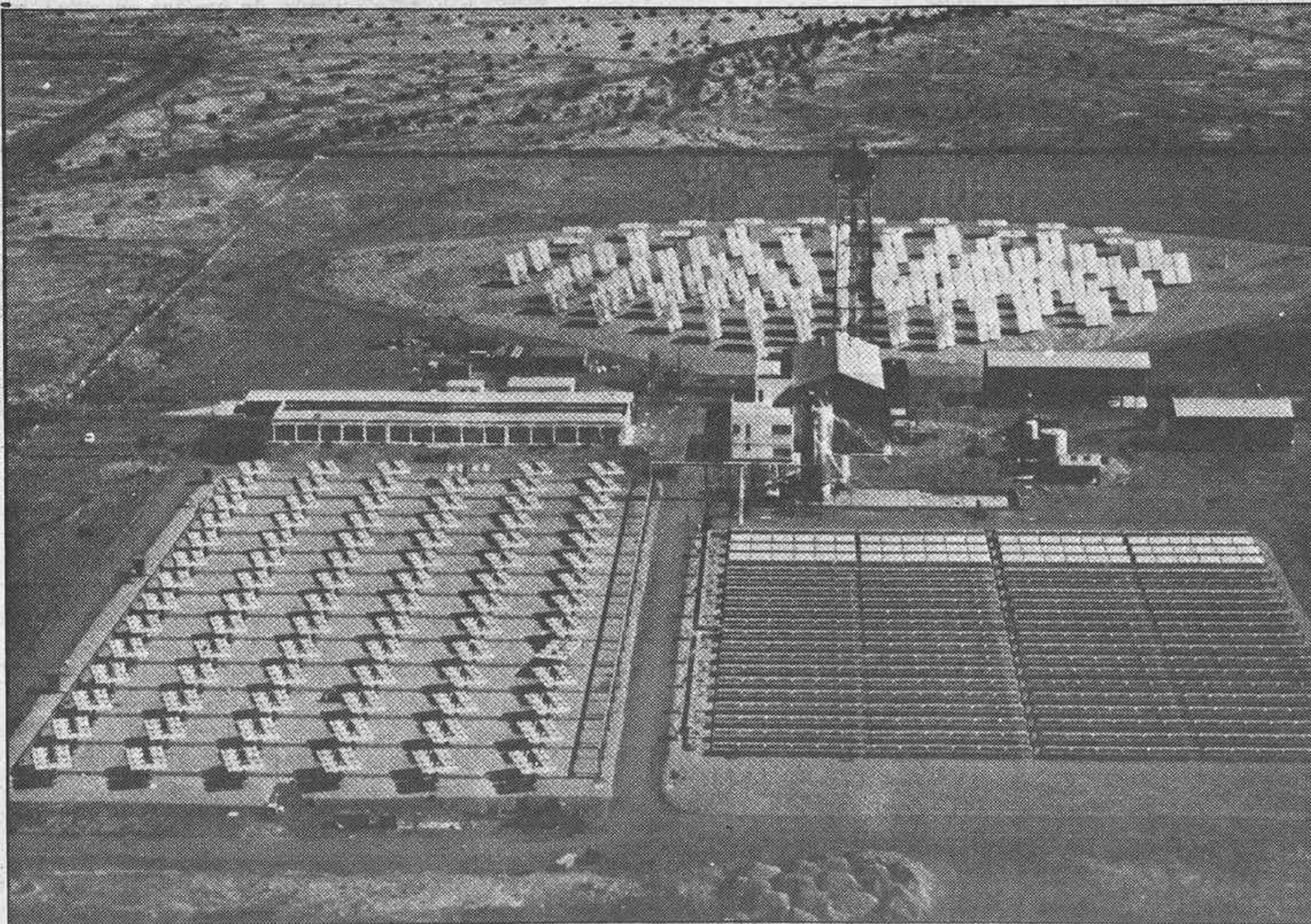
La Central Solar de tipo Torre (en segundo término) construida en Almería por INTERATOM, como contratista general, con una potencia eléctrica de 0,5 MW, está en servicio desde septiembre
