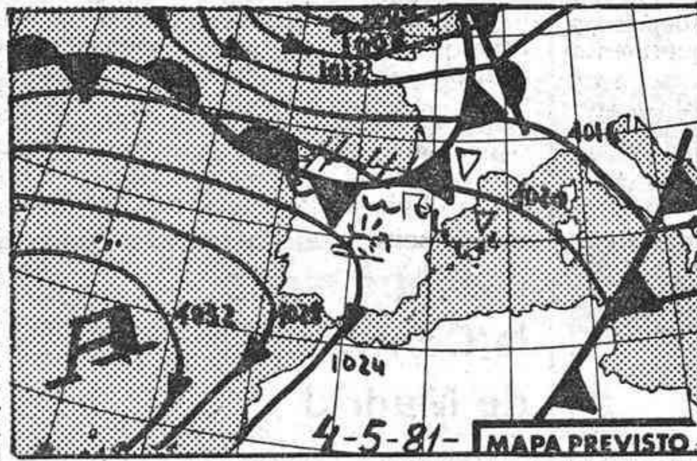
Borrasca en las Islas Británicas y anticiclón al oeste del país, con viento del Norte fresco en las capas altas
