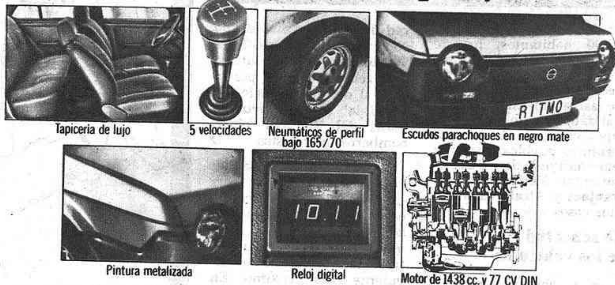
Motor de 1438 cc. y 77 CV DIN
