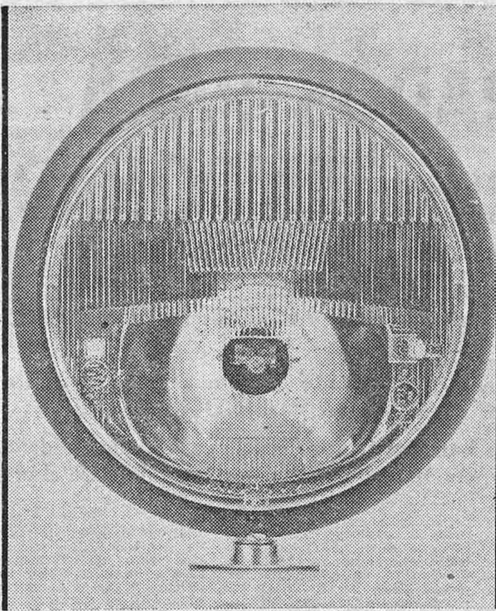
Desde hace quince años, en Francia se conoce el Oscar en dos versiones: antiniebla y largo alcance. Son los ojos actuales de los automóviles. En la versión largo alcance, el cristal de estrias verticales permite obtener un haz de luz confortable, ancho y homogéneo, conservando al tiempo un alcance suficiente. En las luces antiniebla, el cristal dispone de unas estrias particularmente elaboradas que eliminan los rayos autodeslumbrantes y aseguran un haz ancho y gran nitidez
