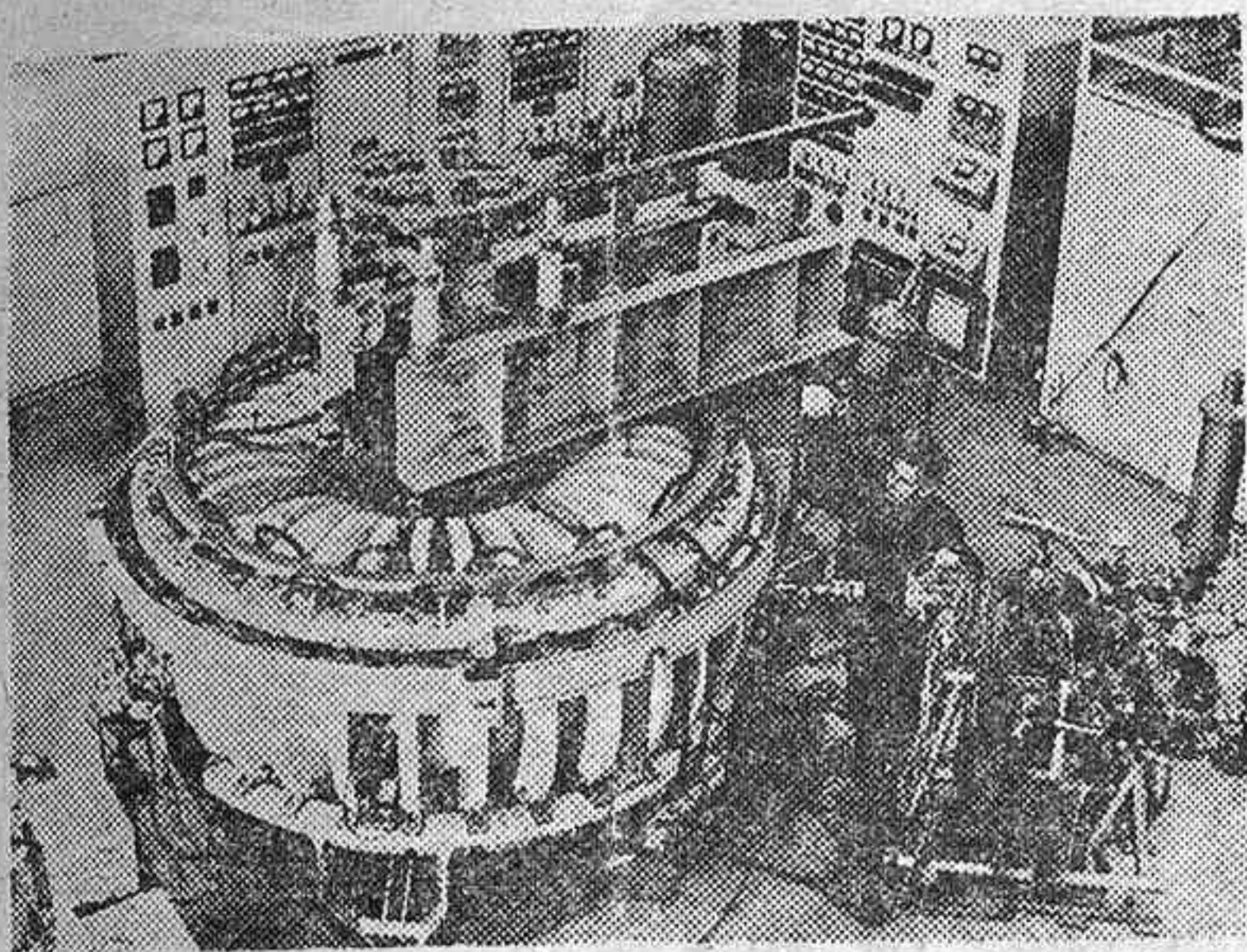
Investigaciones para el desarrollo de un reactor termonuclear controlado
