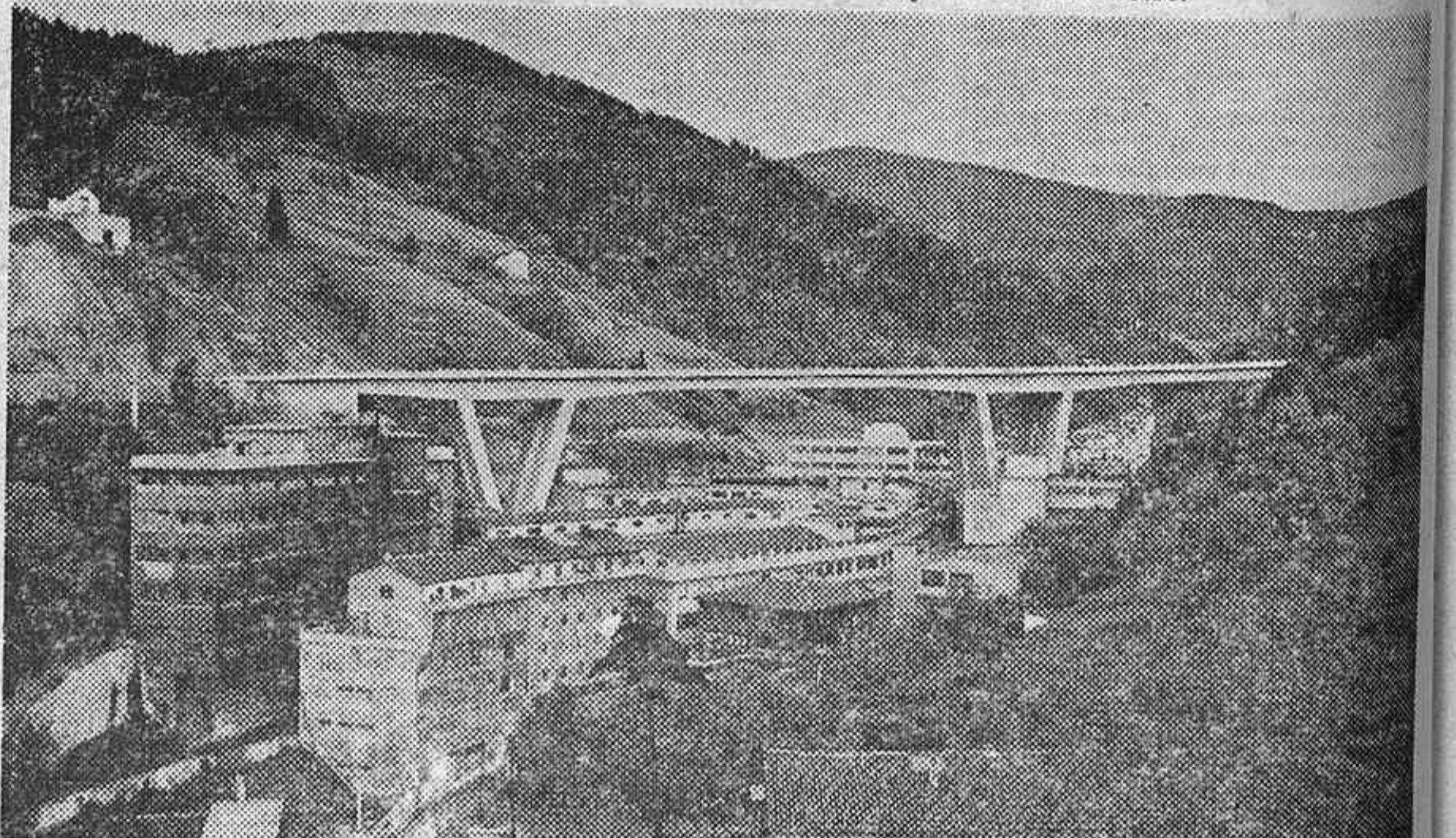
Vista panorámica del viaducto de Chonta, en el tramo Eibar-Elgoibar, de la autopista Bilbao-Irún
