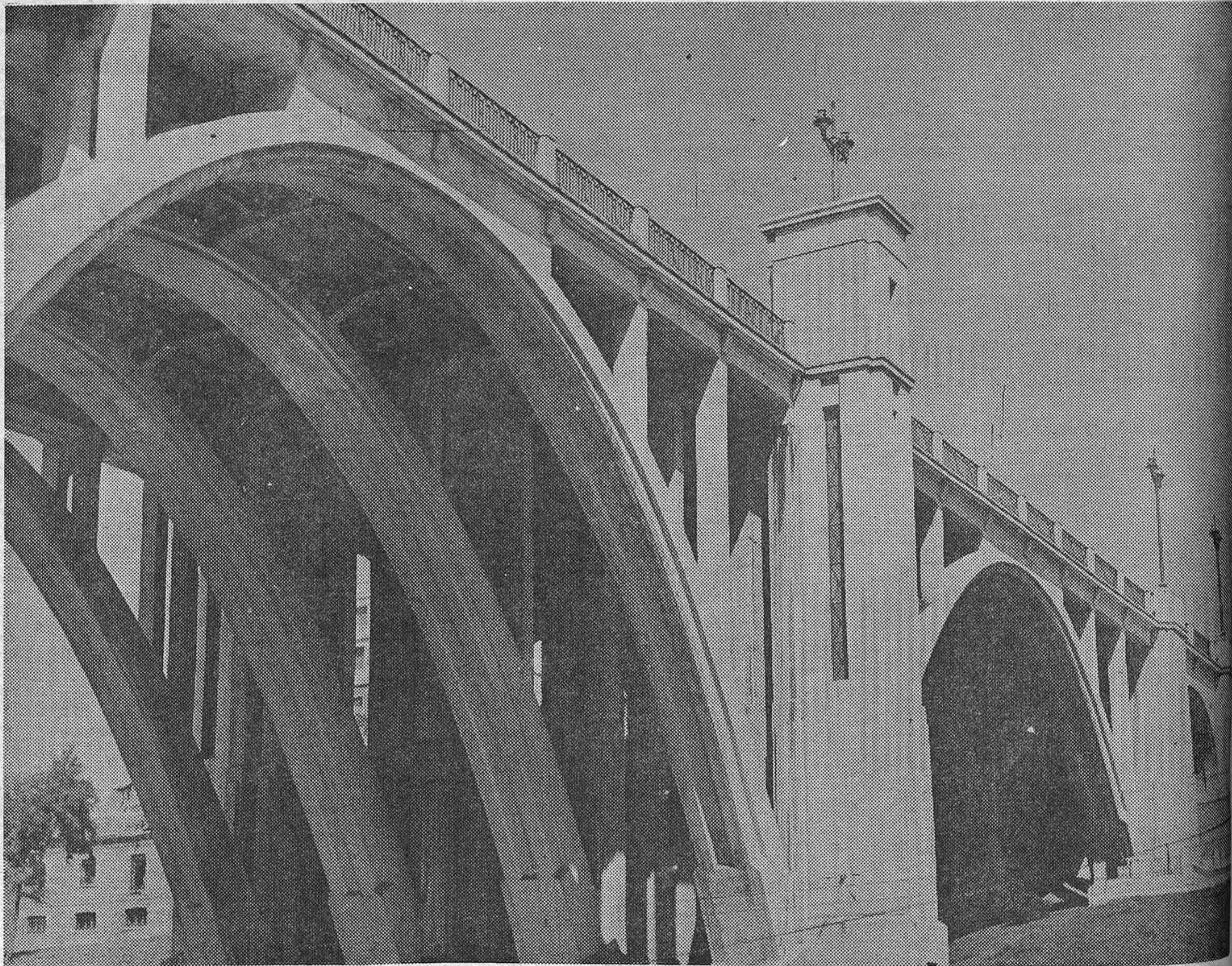
El Viaducto, de cuya posible voladura (?) se habla ahora, ofrece este espléndido espectáculo de equilibrada y funcional arquitectura. El gran pilar central con su sistema de ascensores que salvase en vertical el enorme desnivel entre las calles de Bailén y Segovia. (Foto Torremocha.)
