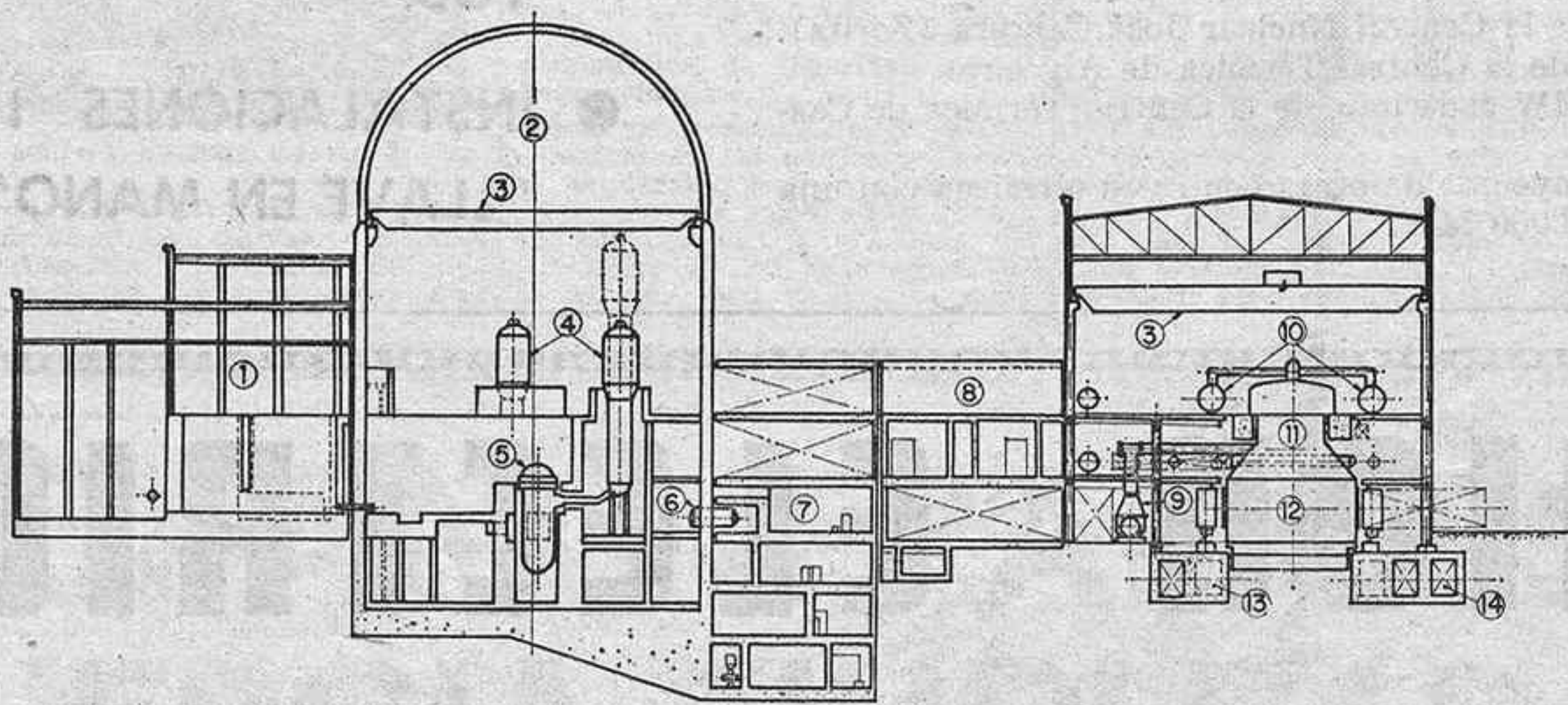
SECCION LONGITUDINAL DE LA CENTRAL
