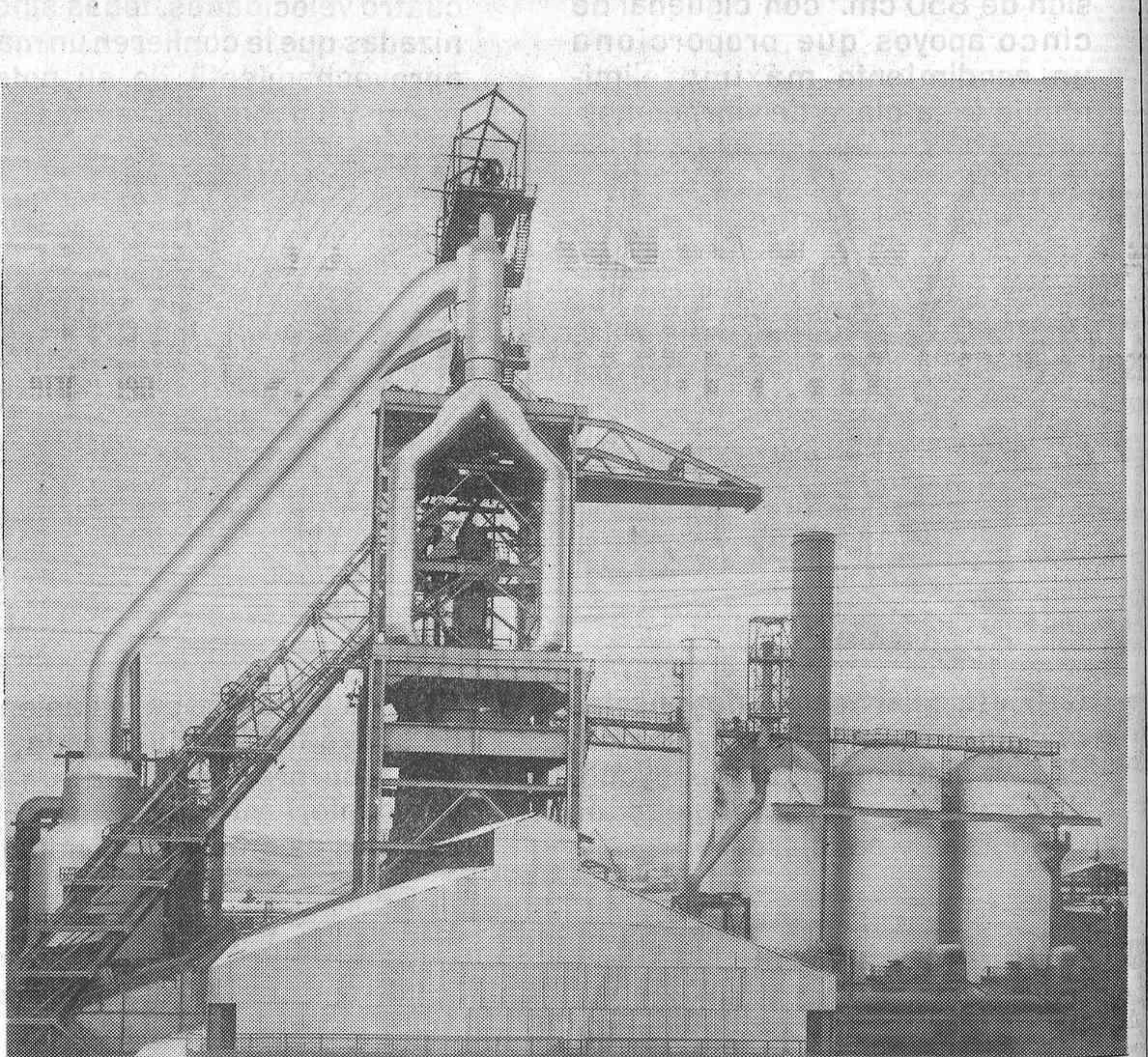
La Industria Siderúrgica española ha incrementado su capacidad de producción al haber puesto en funcionamiento ALTOS HORNOS, en su fábrica de Sestao, el mayor horno alto de España, con una producción diaria de 2.000-3.000 Tn. de arrabio, colocandolo no sólo a la cabeza de los hornos europeos sino incluso a nivel mundial.
