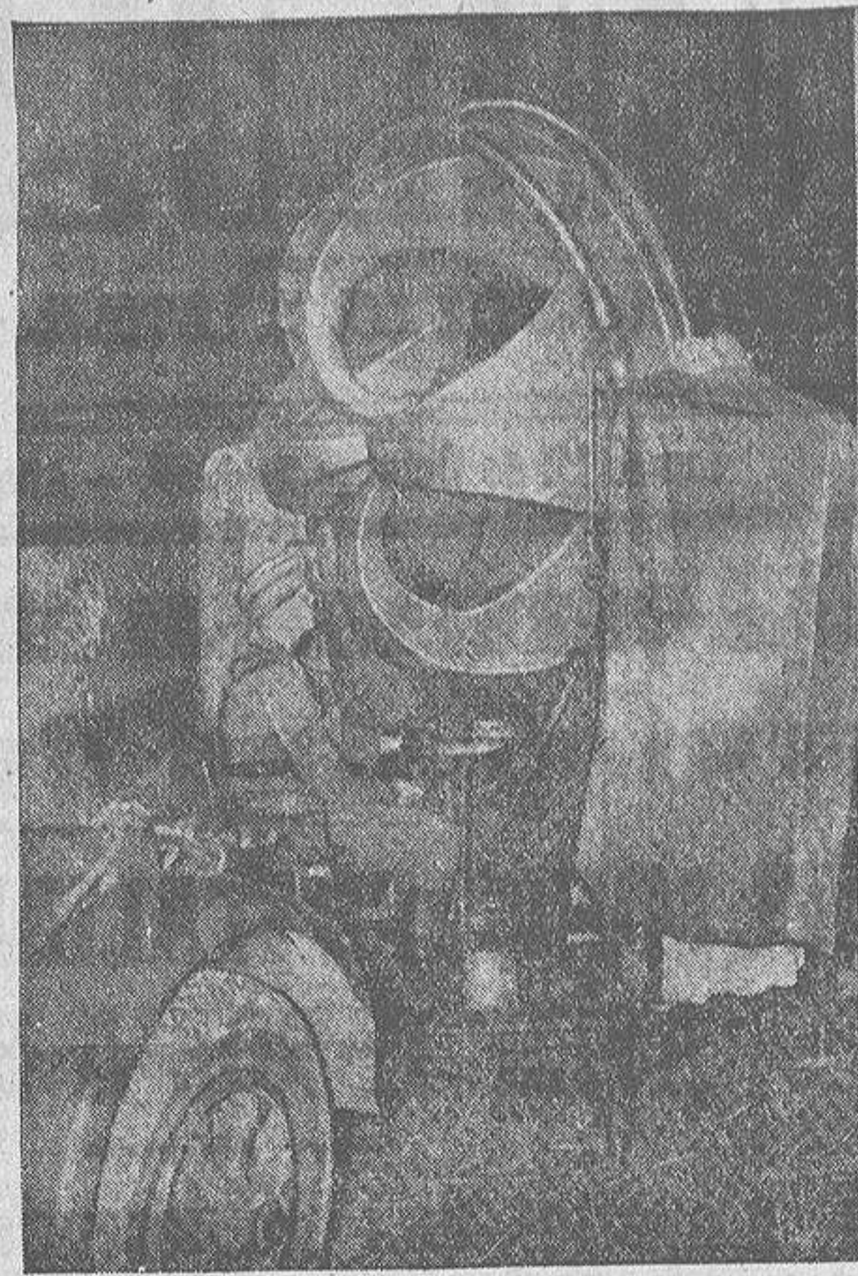
De noche, en la línea Sigfrido, estos aparatos recogen "el rumor del cielo". Es tal el grado de sensibilidad que poseen, que los aviones enemigos son advertidos a treinta kilómetros de distancia.
