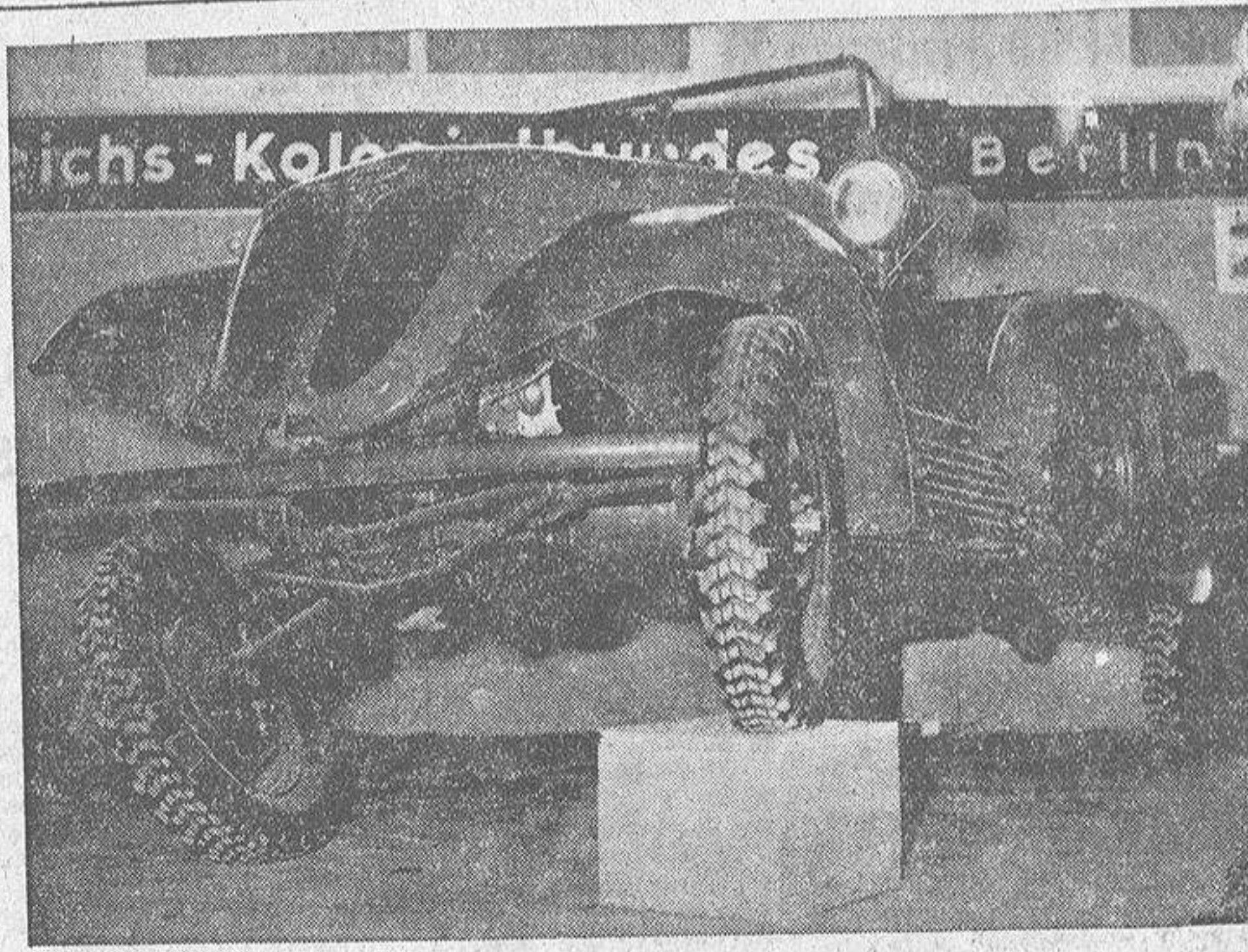
Feria de Primavera en Leipzig 1939. Coche-modelo "Tempo". Un automóvil ideal para toda clase de terrenos, apropiado para regiones de la zona tropical y de ultramar. La adaptación a terreno accidentado es sorprendente, y esto a causa de la construcción especial del coche.
