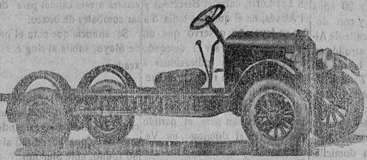
CHASSIS *RUGBY, 4 CILINDROS 1 1/2 y 1 1/2 TONELADAS
