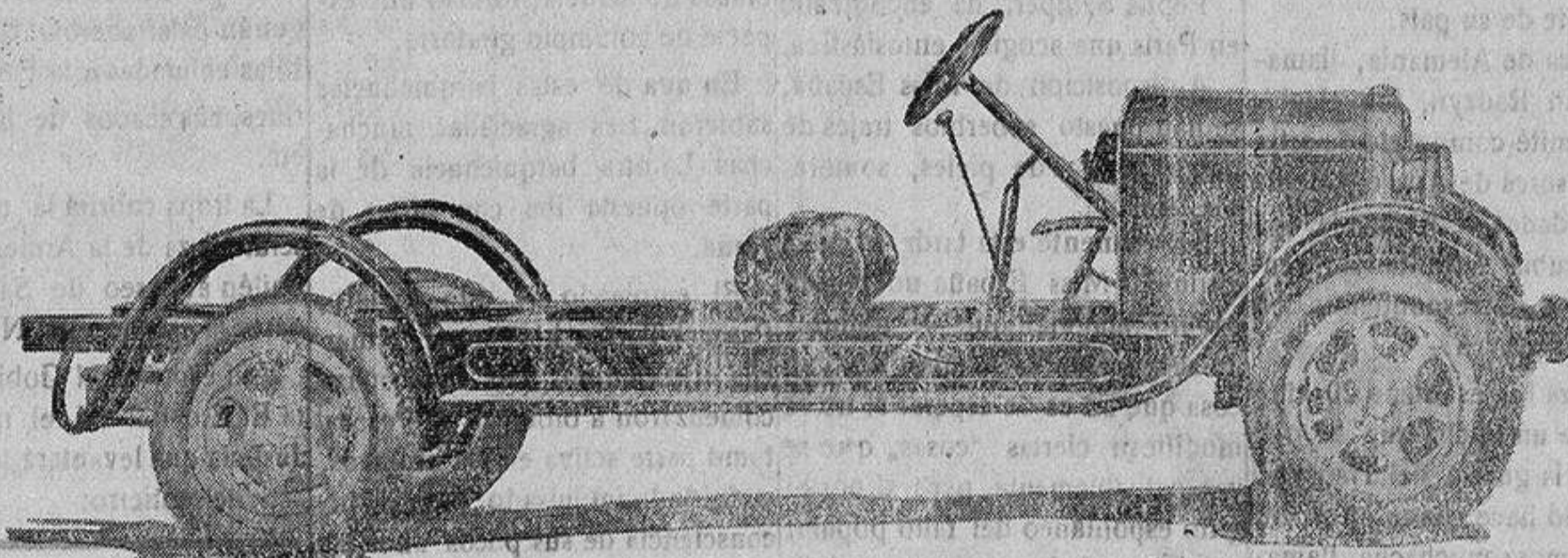
CHASSIS "RUGBY", 6 CILINDROS. 2 TONELADAS Con doble directa, (cuatro velocidades)
