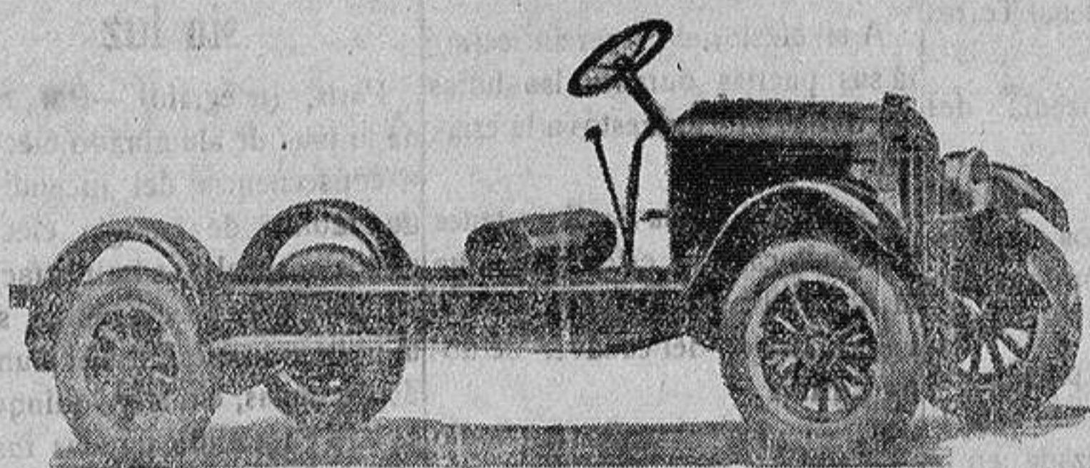
CHASSIS "RUGBY", 4 CILINDROS 1 y 1/2 TONELADAS
