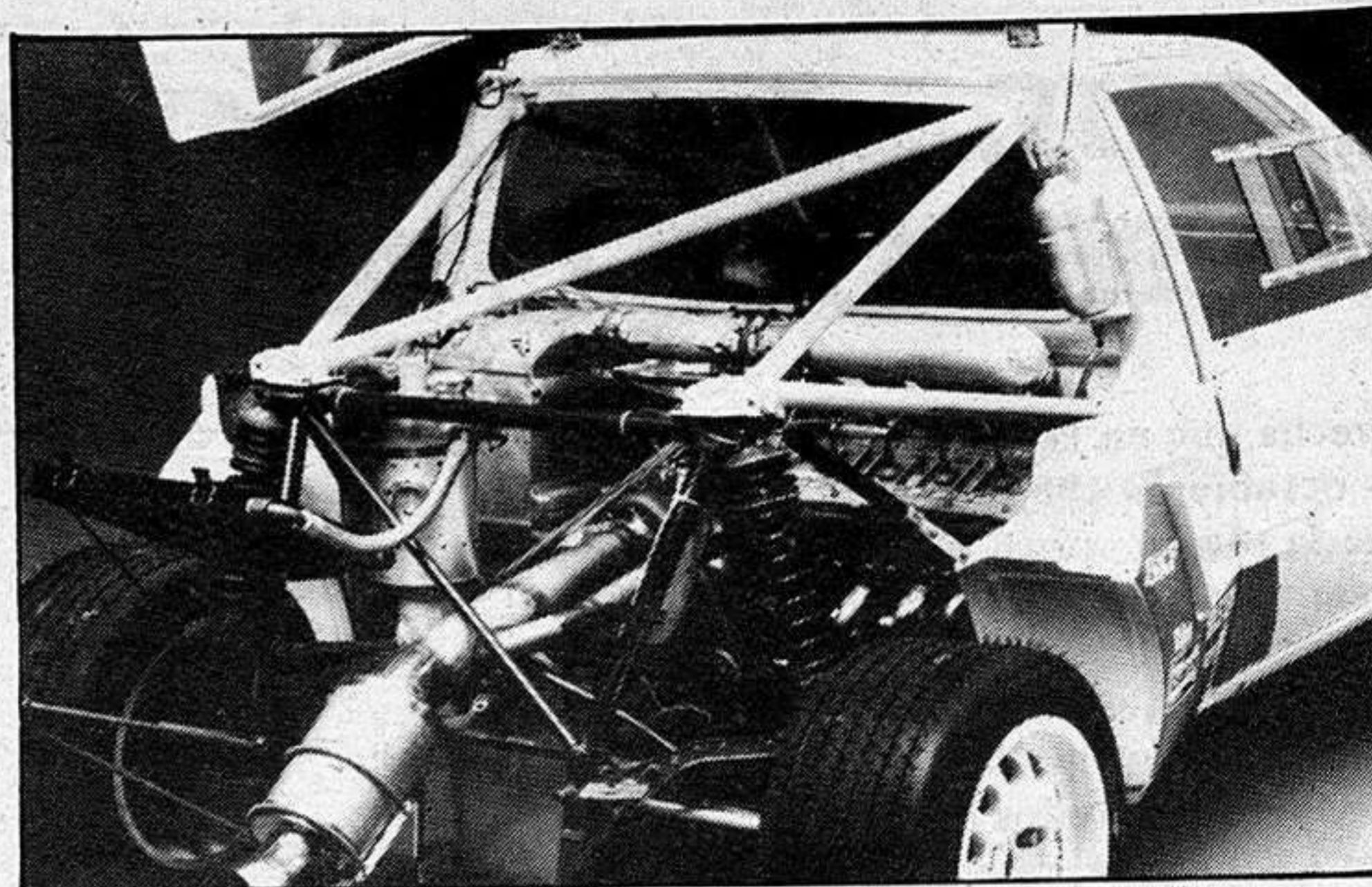
Una nueva culata y un turbocompresor Garret con una presión máxima de 2,5 bares, han logrado que la potencia del motor, que respeta las cotas generales del anterior, ascienda a 430 CV
