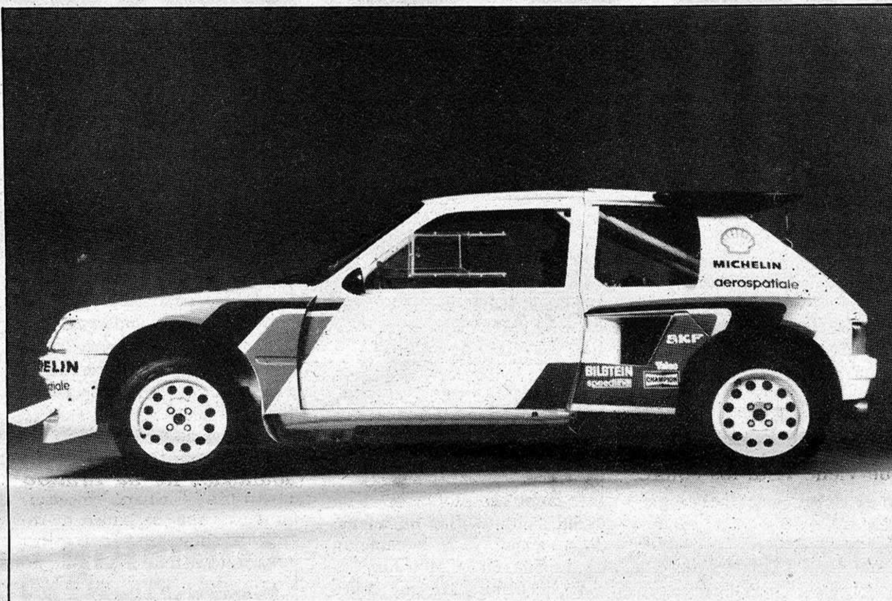
El Peugeot 205 Turbo 16 "Evolución 2" se caracteriza por la adopción de spoiler y alerones muy prominentes. El spoiler delantero está equipado de una mánina móvil
